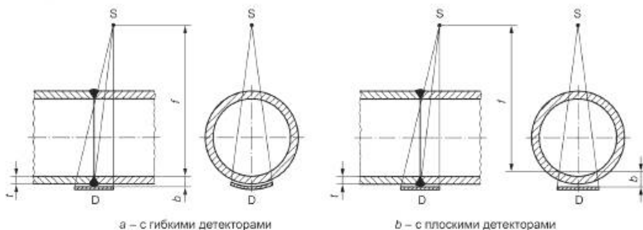
Рисунок 13 — Схема контроля изогнутых объектов при просвечивании через две стенки (одно изображение) для контроля стенки, ближайшей к детектору: |Q| располагается на детекторе
