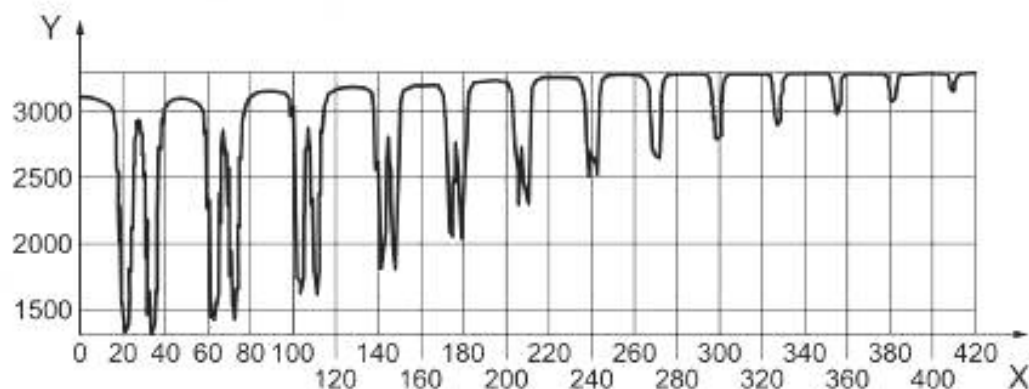
б — Профиль IQI двухпроводочного типа, усредненный, как минимум, по 21 линии
