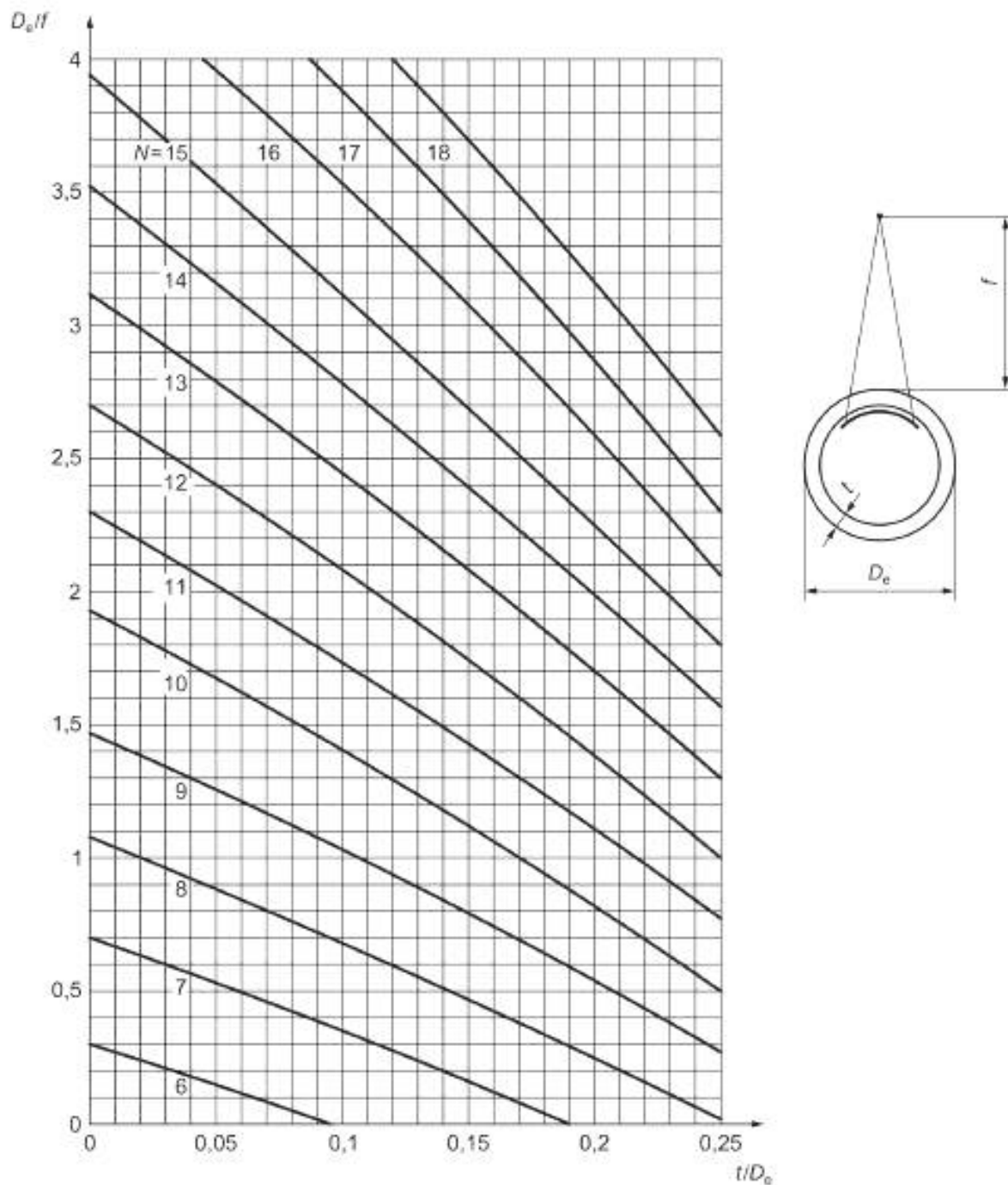
Рисунок А.3 — Минимальное количество экспозиций N при просвечивании через одну стенку с источником излучения снаружи при максимально допустимом увеличении просвечиваемой толщины \Delta t/f из-за наклонного направления излучения в проверяемой области, равном 20 % (класс А), как функция отношений t/D_e и D_e/f
