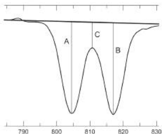
д — Схема расчета отношения глубины впадины к пикам на профиле распределения значений градаций серого (dip): \text{dip} = 100 \cdot (A + B - 2C) / (A + B), \%
