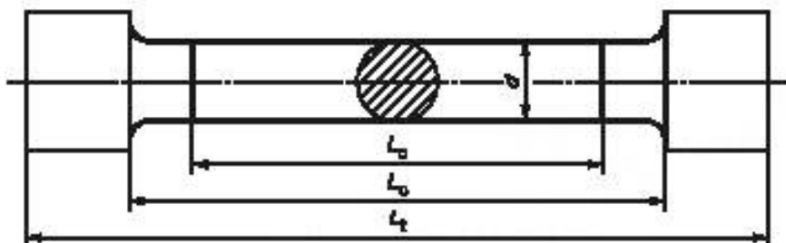
Рисунок 3 — Образец для испытания на растяжение металла шва
