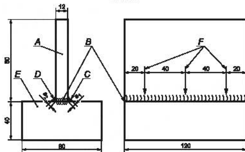
a — толщина шва (6 мм); A — вертикальный лист; B — прихваточные швы; C — сварной шов 1; D — сварной шов 2; E — горизонтальный лист; F — места измерения
