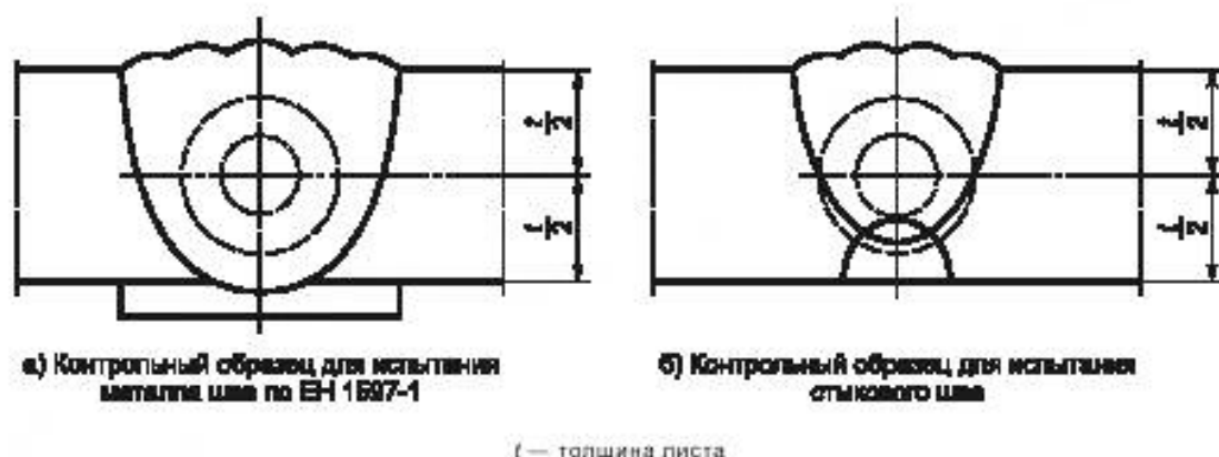
Рисунок 2 — Изготовление из контрольных образцов для испытания на растяжение металла шва
