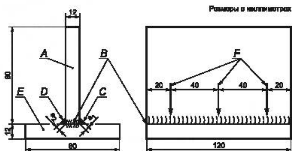
A — вертикальный лист; B — прихваточные швы; C — сварной шов 1; D — сварной шов 2; E — горизонтальный лист; F — места измерения
