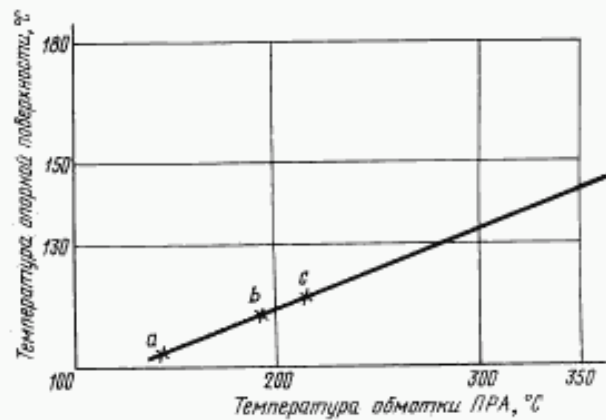
a, b, c — измеренные значения температуры при 0,9-, 1,0 и 1,1-кратном номинальном напряжении
