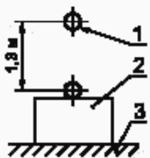
1 — стальной шарик; 2 — светильник; 3 — опорная поверхность
