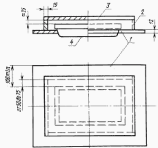
1 — основа, 2 — боковая стенка, 3 — верхняя стенка, 4 — испытуемый светильник
