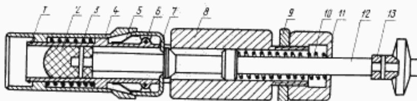
1 — кольцо стопорное; 2 — наконечник; 3 — пружина; 4 — головка; 5 — пружина; 6 — ось; 7 — фиксатор; 8 — корпус; 9 — гайка; 10 — пружина; 11 — колпачок; 12 — шток; 13 — ручка
