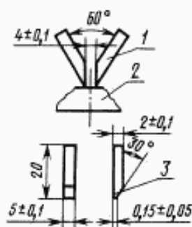
1 — электрод; 2 — испытуемый образец; 3 — конец электрода скруглен
