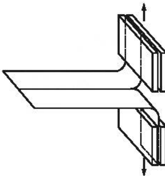
Рисунок 3 — Метод крепления образца для испытаний в зажимах
