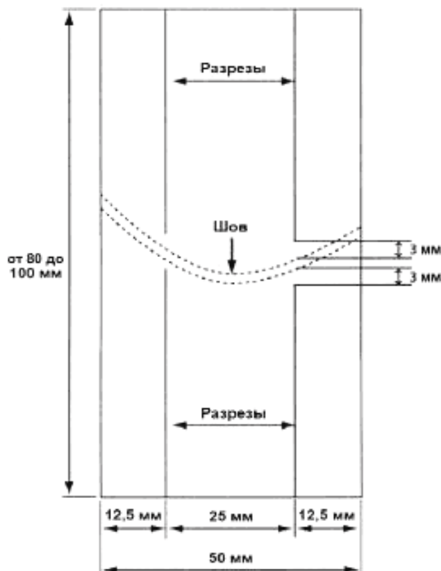
Рисунок 3 — Образец, вырезанный из готового изделия
