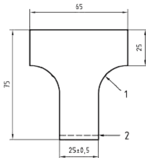
Рисунок 2 — Образец для испытания
