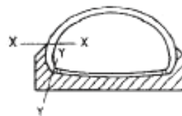
Тип d: Затыжка Strobel Клеевая формованная подошва, прямой впрыск или вулканизация подошвы
