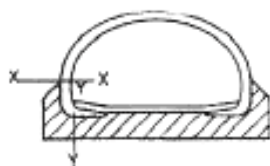
Тип с: Стандартная затыжка Прямой впрыск или вулканизация подошвы или клеевая формованная подошва
