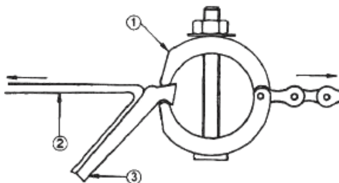
1 – зажим для короткого края подошвы; 2 – верх; 3 – подошва
