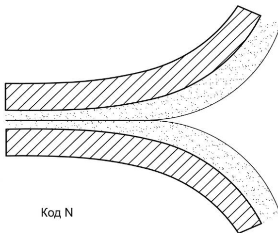
Рисунок 8 — Недостаточная коалесценция
