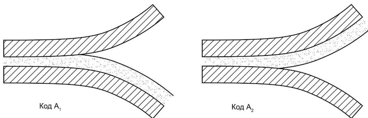
Рисунок 6 — Недостаточная адгезия
