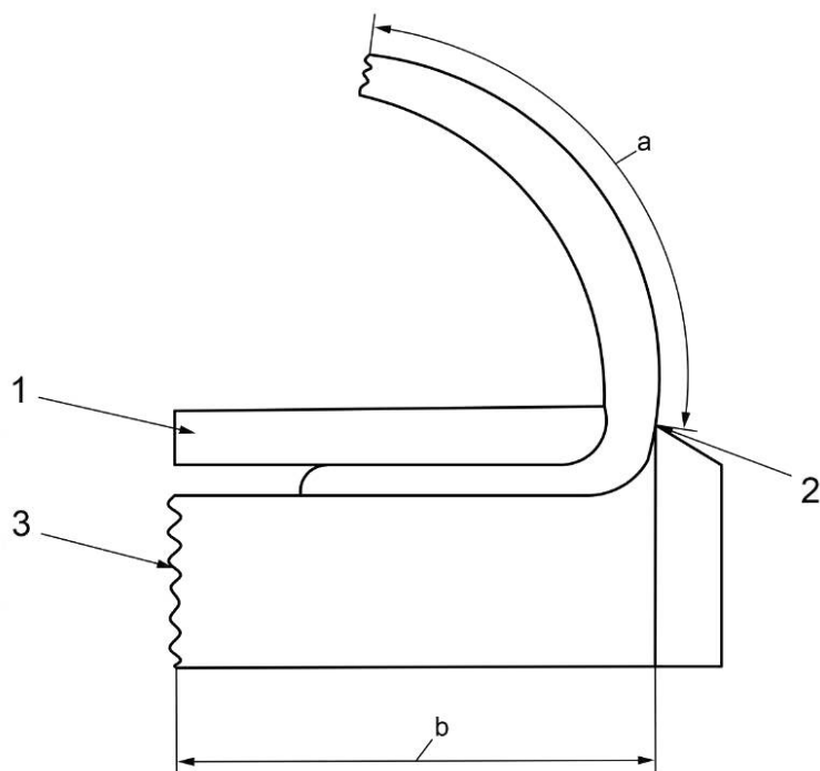
Рисунок 2 — Поперечное сечение испытуемого образца
