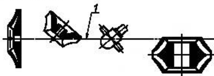
1 — Базовая плоскость NPSH
