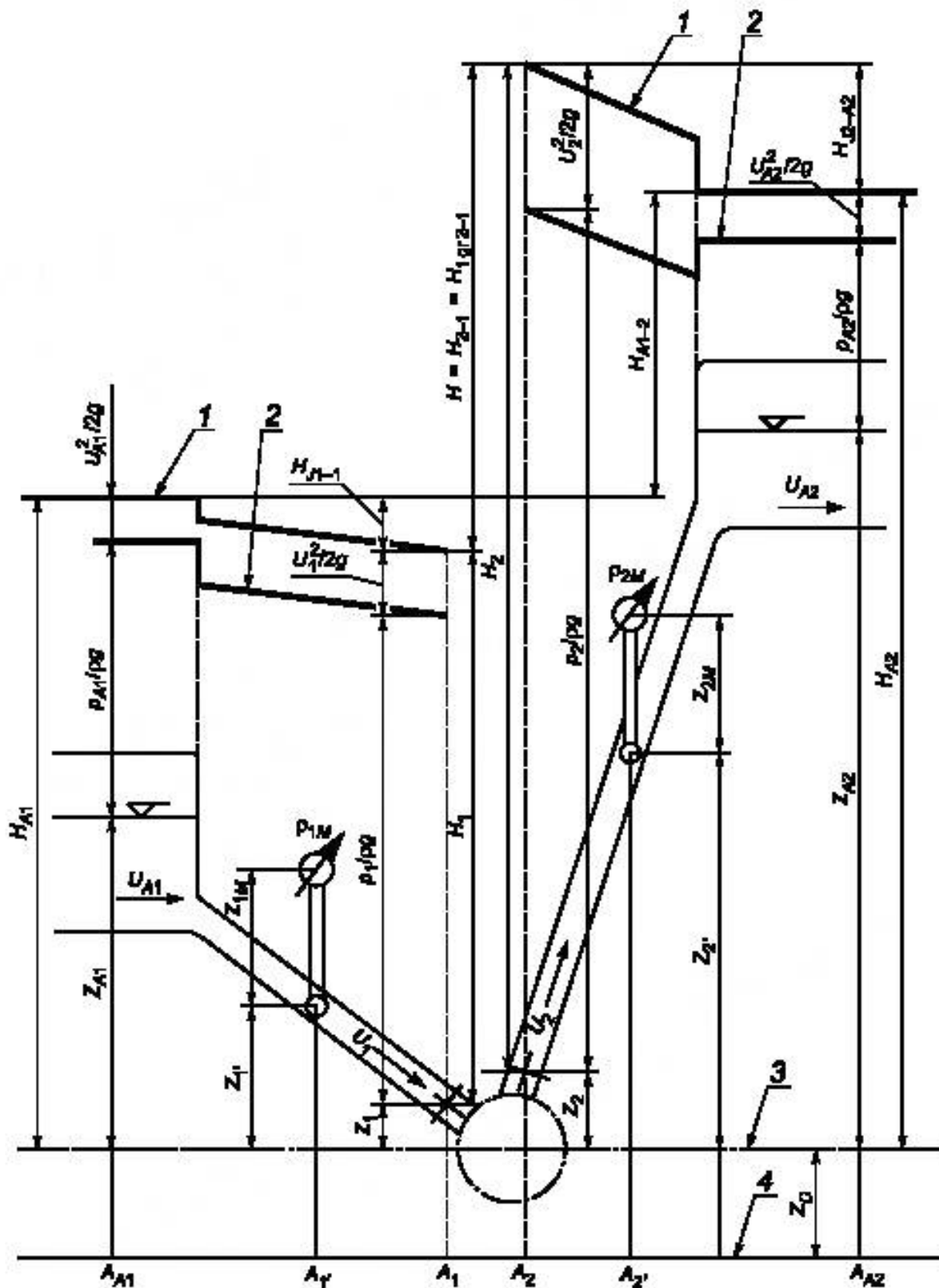
Рисунок А.1, лист 1 — Определение полного напора насоса
