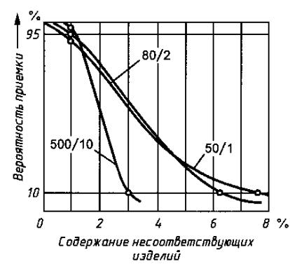
Кривые оперативных характеристик для планов выборочного контроля
