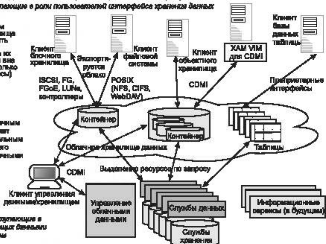
Рисунок 3 – Эталонная модель облачного хранилища
