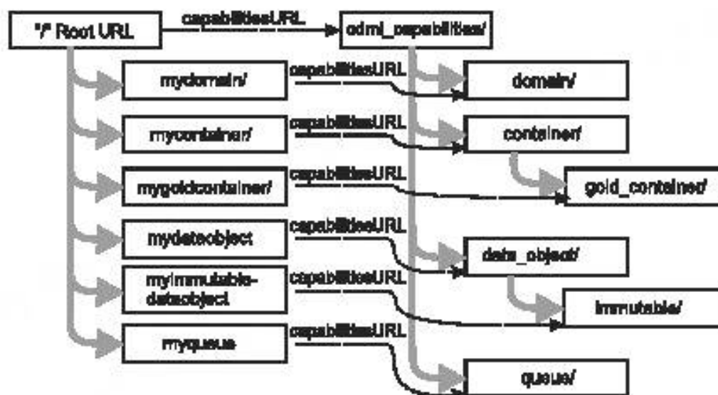
Рисунок 7 – Иерархия опций
