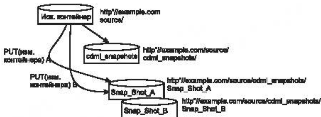
Рисунок 9 – Структура снимка состояния контейнера
