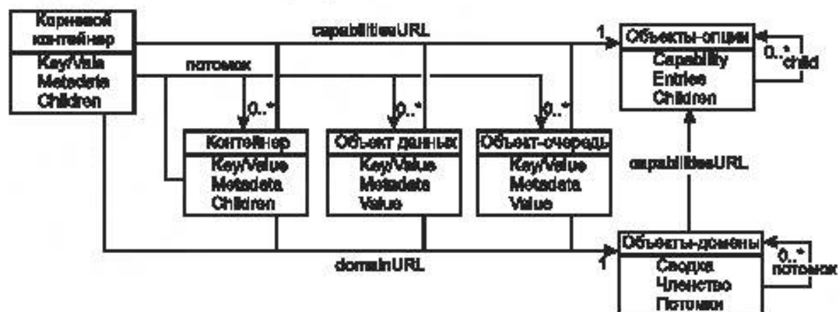
Рисунок 4 – Модель объекта CDMI
