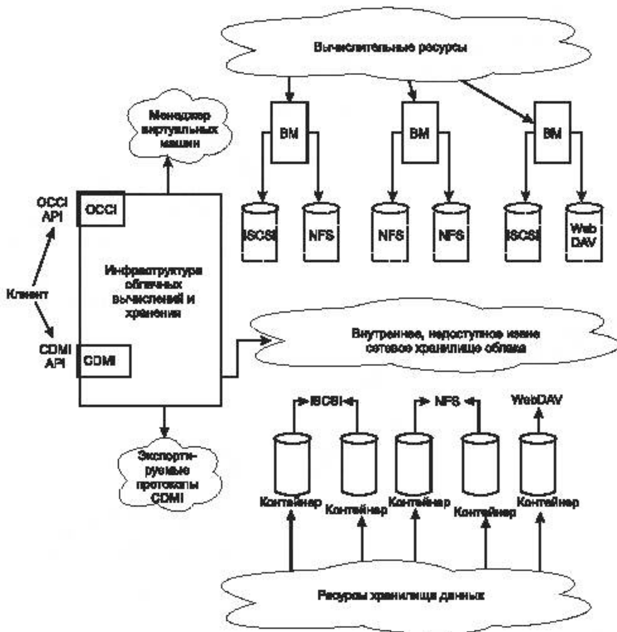
Рисунок 8 – CDMI и OCCI в интегрированной облачной вычислительной среде
