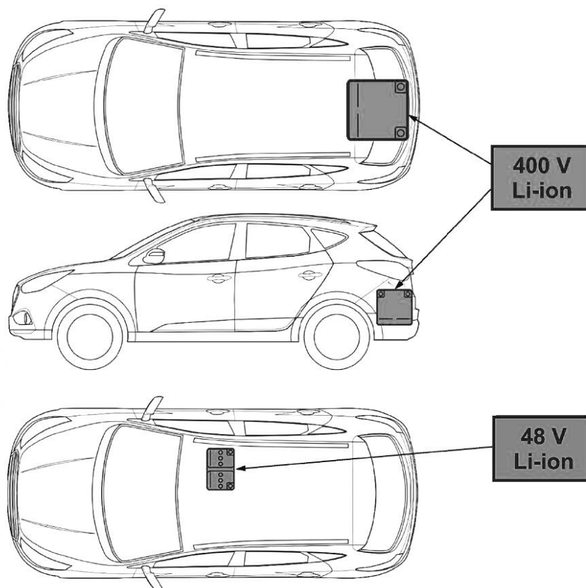
Рисунок 2 — Напряжение аккумулятора и индикатор технологии
