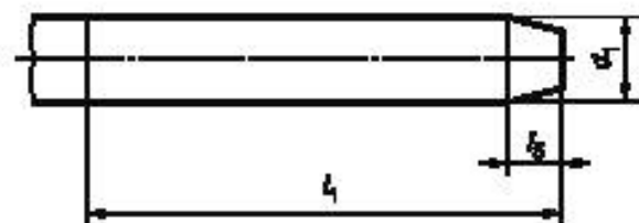
Рисунок 4 — Хвостовик типа 3
