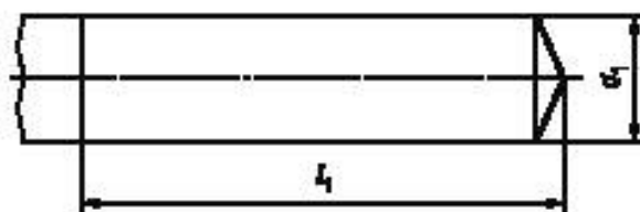
Рисунок 3 — Хвостовики типа 2 и типа 4
