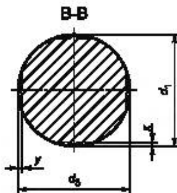
Рисунок 10 — Сплющивание участков, поперечное сечение В-В на рисунке 9
