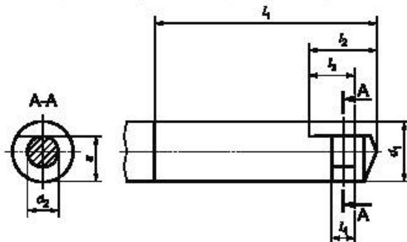
Рисунок 2 — Хвостовик типа 1
