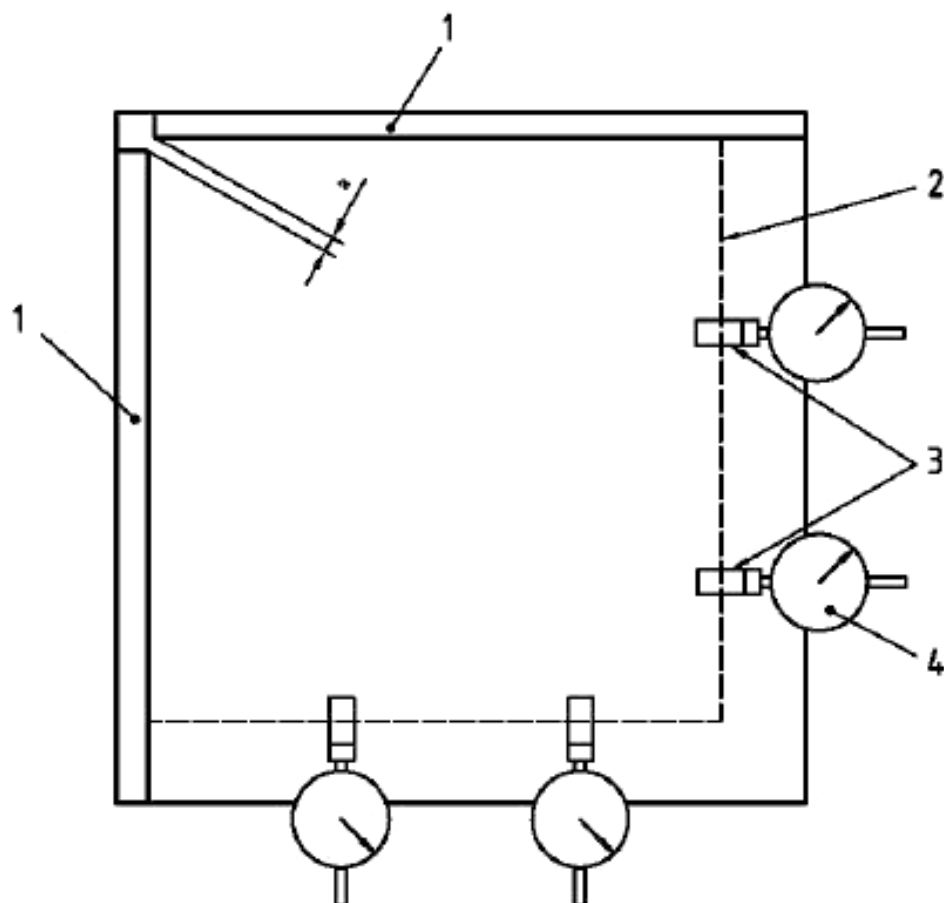
1 — упоры; 2 — образец; 3 — пазы/прорези; 4 — микрометры a Приблизительно 1 мм.
