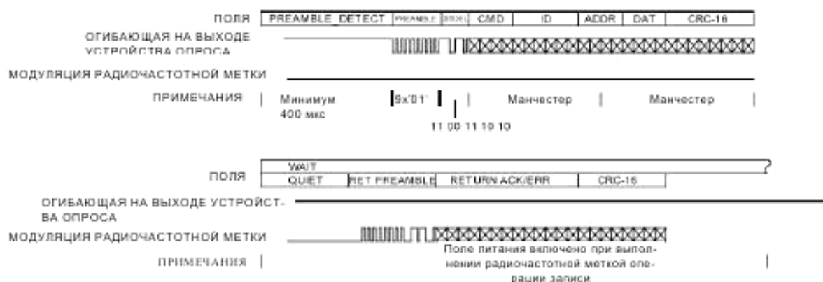
Рисунок 13 — Пример пакетов команды WRITE
