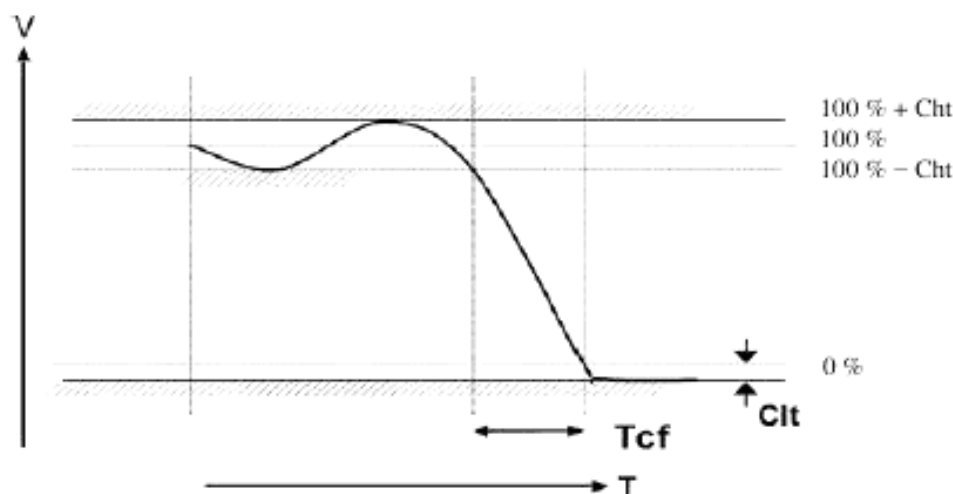
Рисунок 2 – Форма огибающей сигнала при выключении устройства опроса
