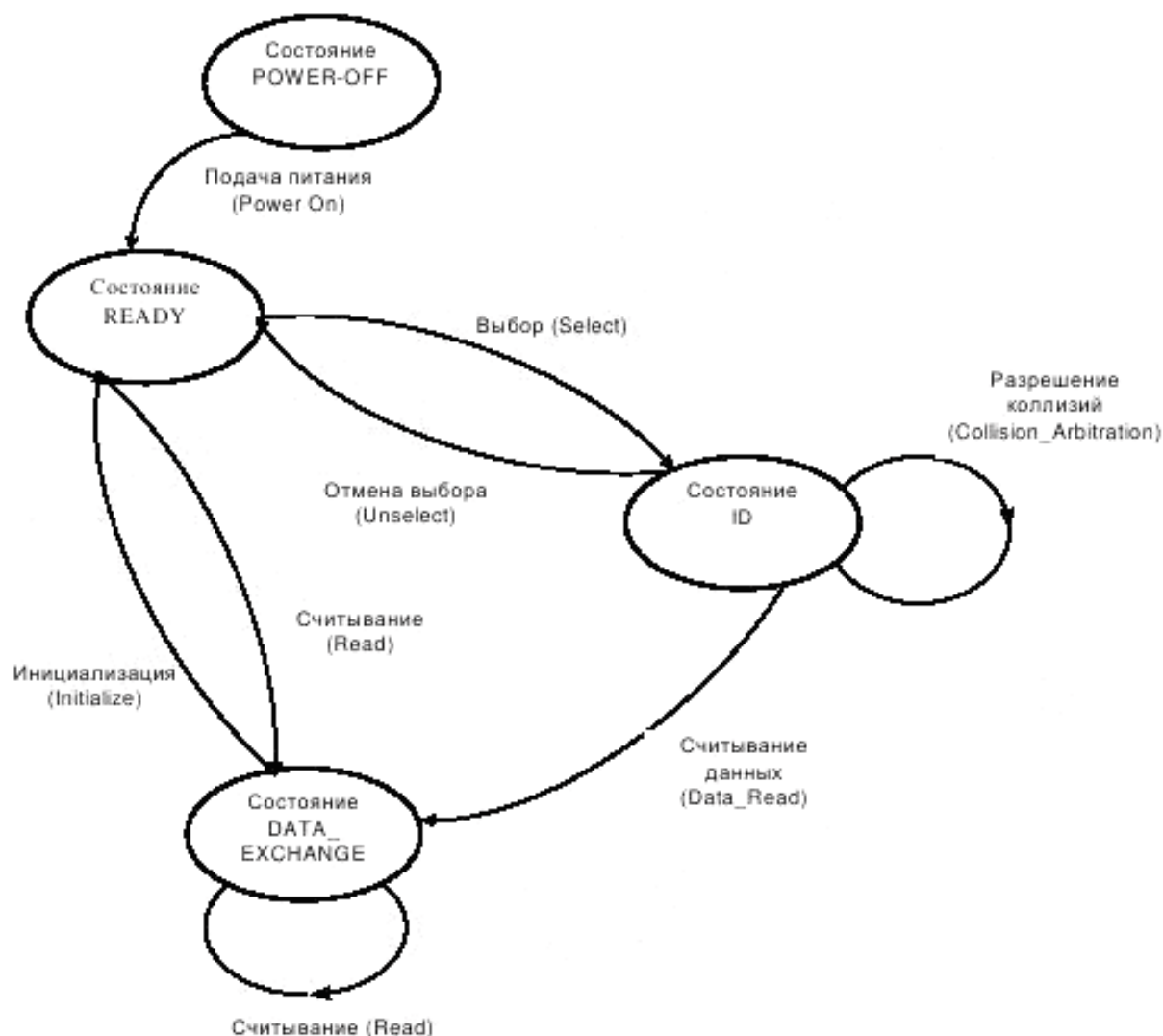
Рисунок 16 – Диаграмма состояний
