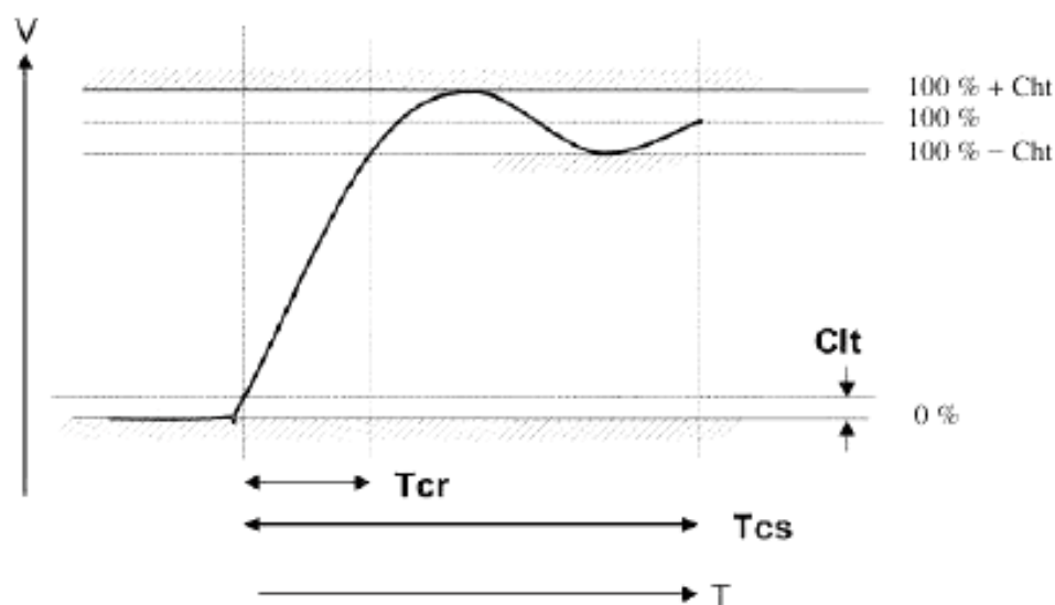
Рисунок 1 – Форма сигнала при включении устройства опроса
