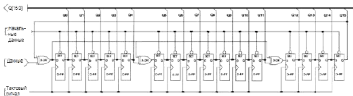
Рисунок А.1 – Пример схемы контроля кодом CRC-16
