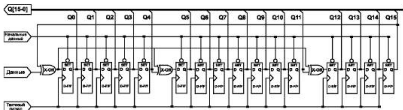
Рисунок А.1 — Пример схемы контроля кодом CRC-16
