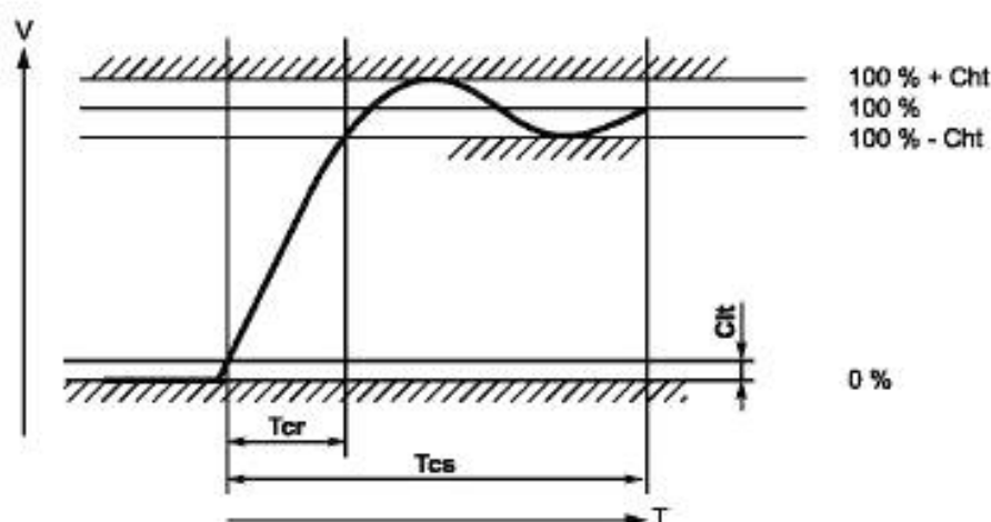
Рисунок 1 — Форма сигнала при включении устройства опроса
