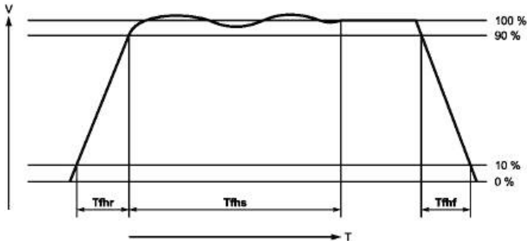
Рисунок 3 — Характеристики нарастания и спада несущей в режиме FHSS
