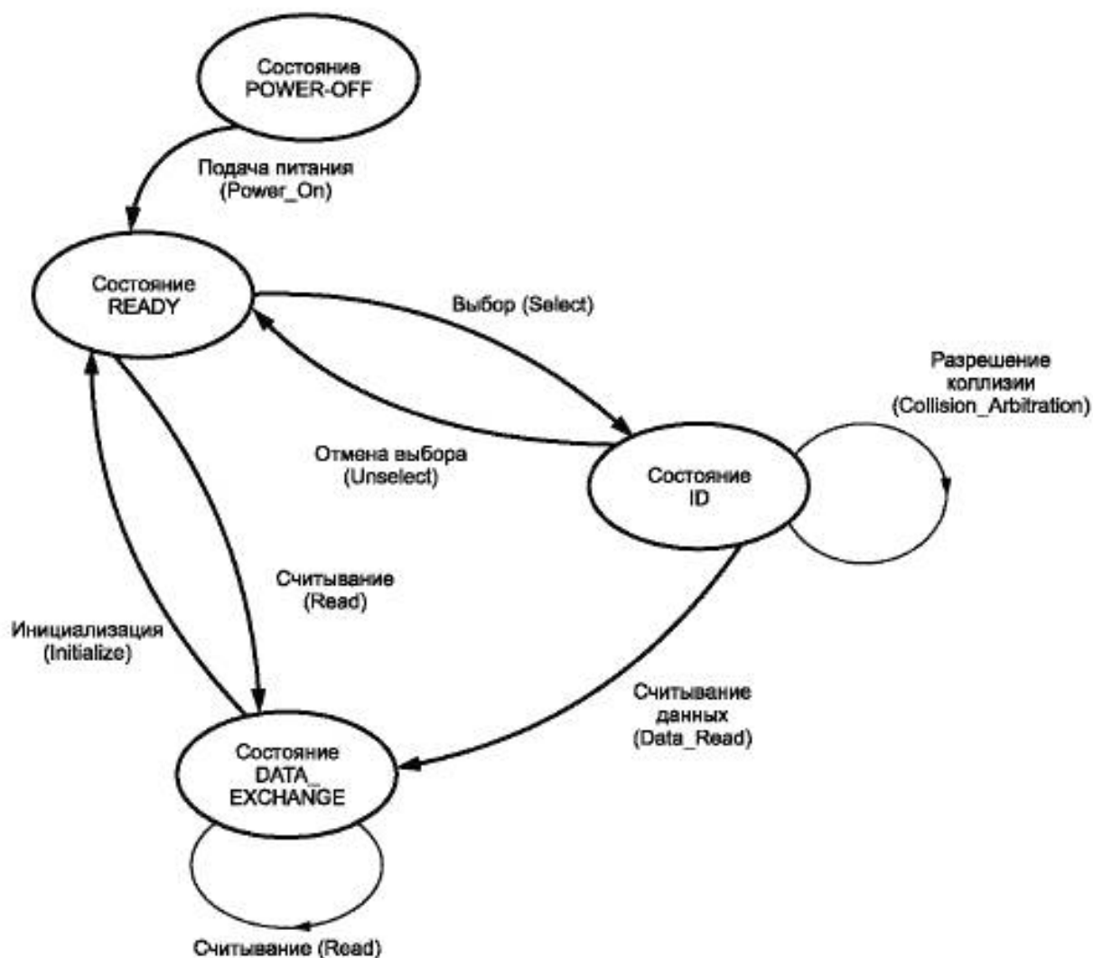
Рисунок 16 — Диаграмма состояний
