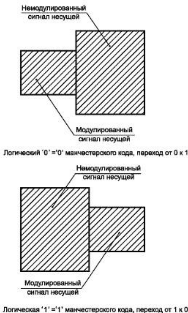
Рисунок 9 — Кодирование бита данных в прямой линии связи
