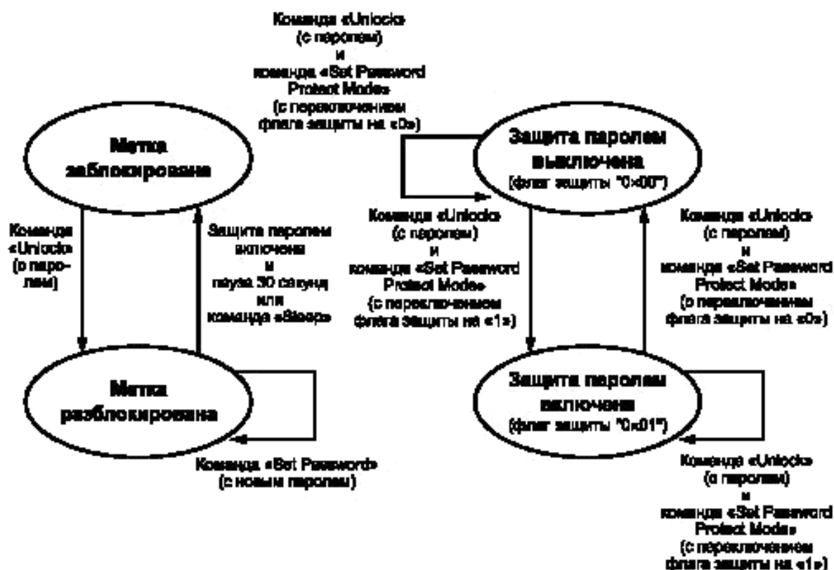
Рисунок 4 — Схема состояний механизма защиты
