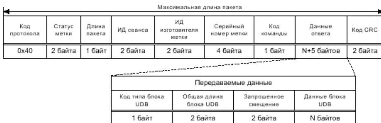
Рисунок 9 — Ответ радиочастотной метки на команду «Collection with UDB»
