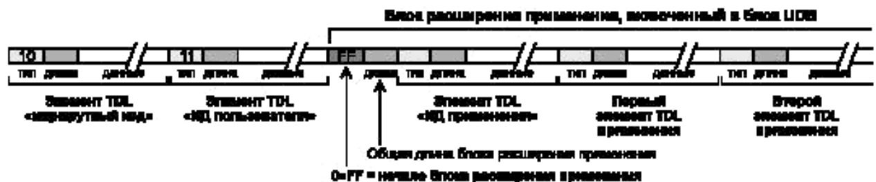
Рисунок 3 — Пример универсального блока данных (блока UDB) типа 0x00
