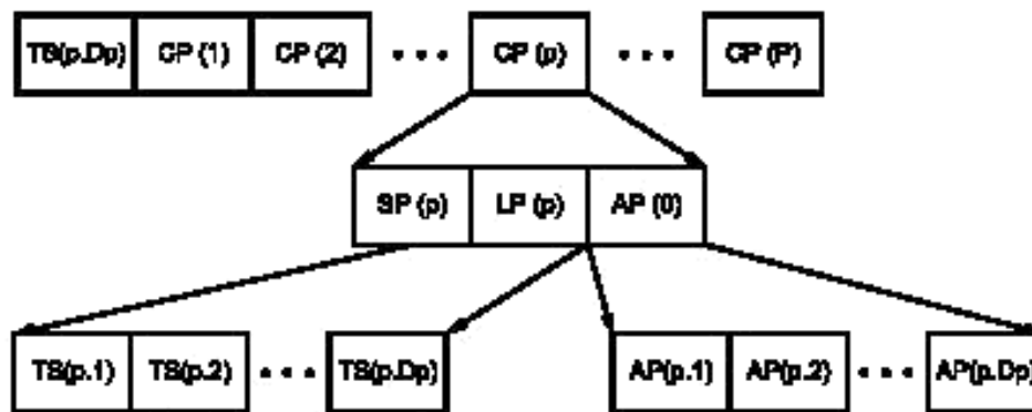
Рисунок 6 — Подробная диаграмма синхронизации антиколлизийного алгоритма
