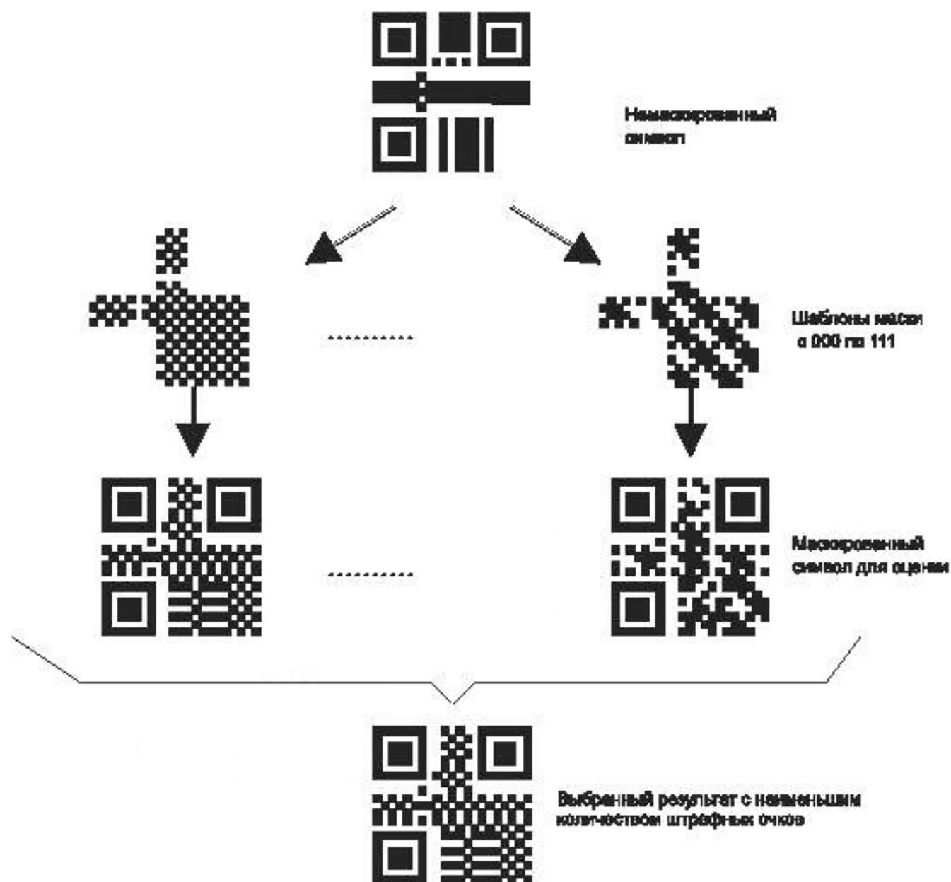
Рисунок 23 – Пример маскирования данных в символах QR Code
