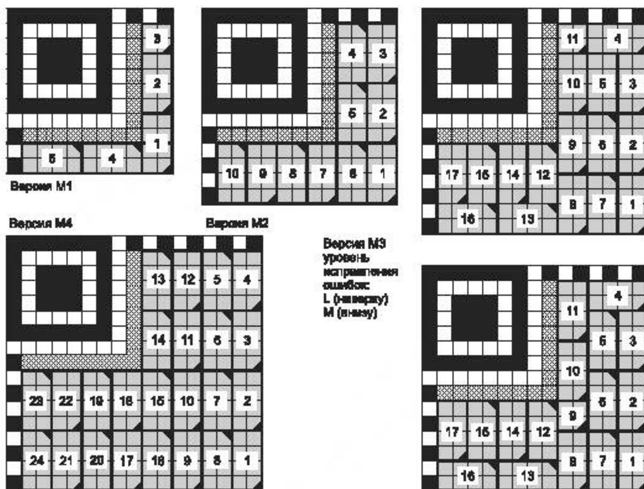
Рисунок 11 — Версии символов Micro QR Code
