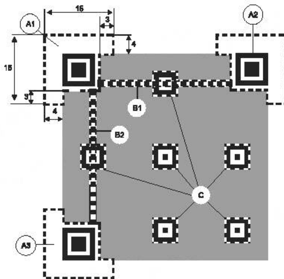
Рисунок G.1 — Сегменты фиксированного шаблона QR Code
