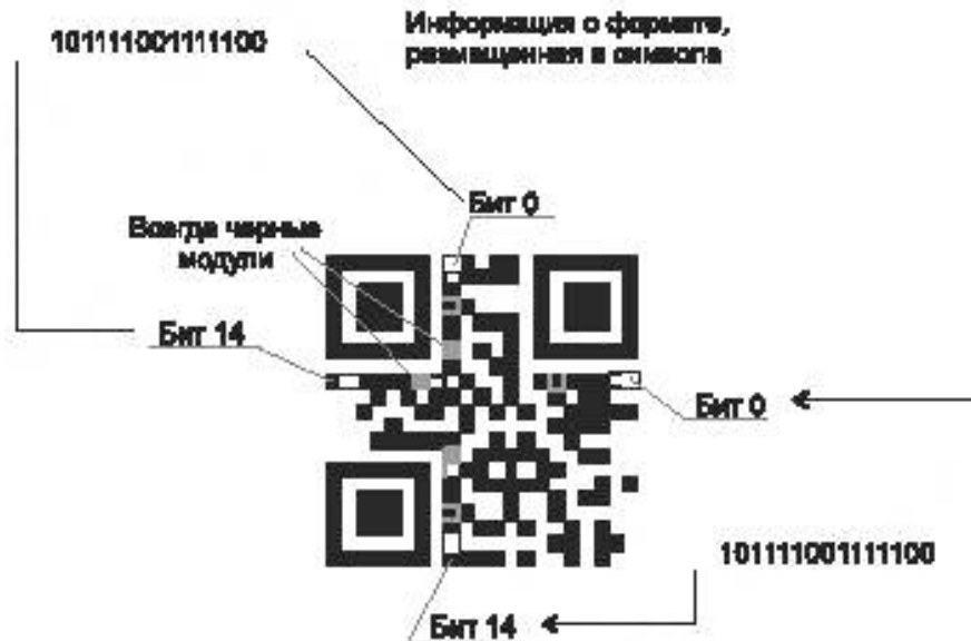
Рисунок I.2 — Окончательный вид символа версии 1-M, кодирующего 01234567
