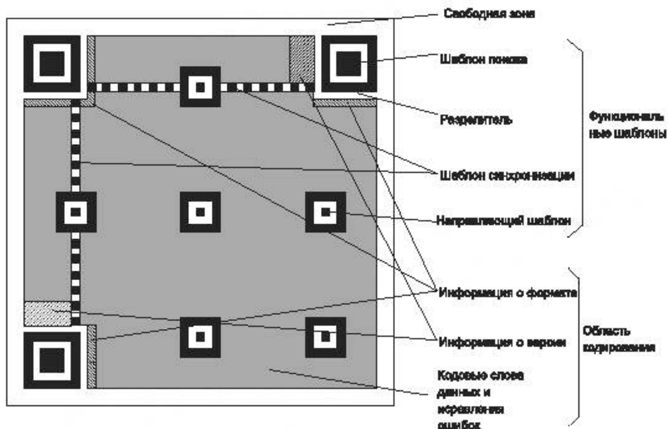
Рисунок 3 — Структура символа QR Code версии 7
