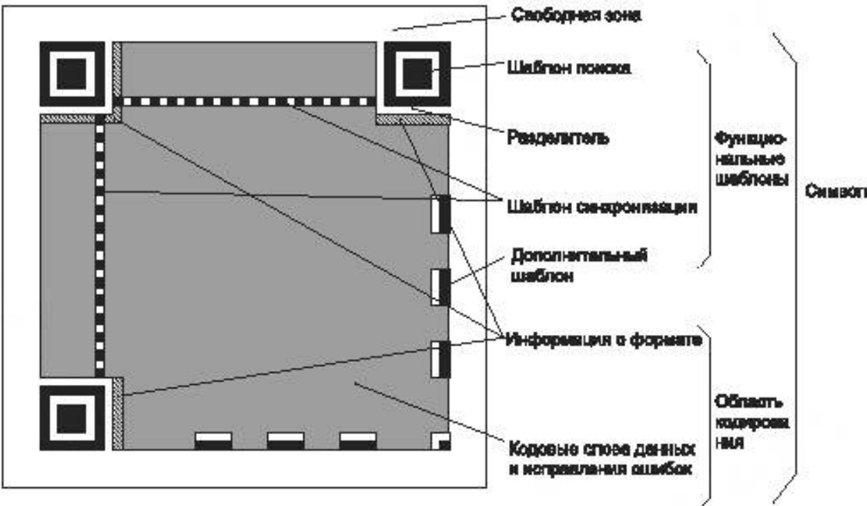
Рисунок N.1 — Структура символа QR Code Model 1
