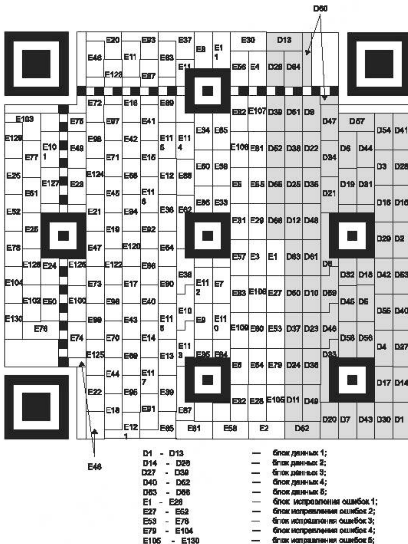
Рисунок 20 – Размещение знаков символа версии 7-H
