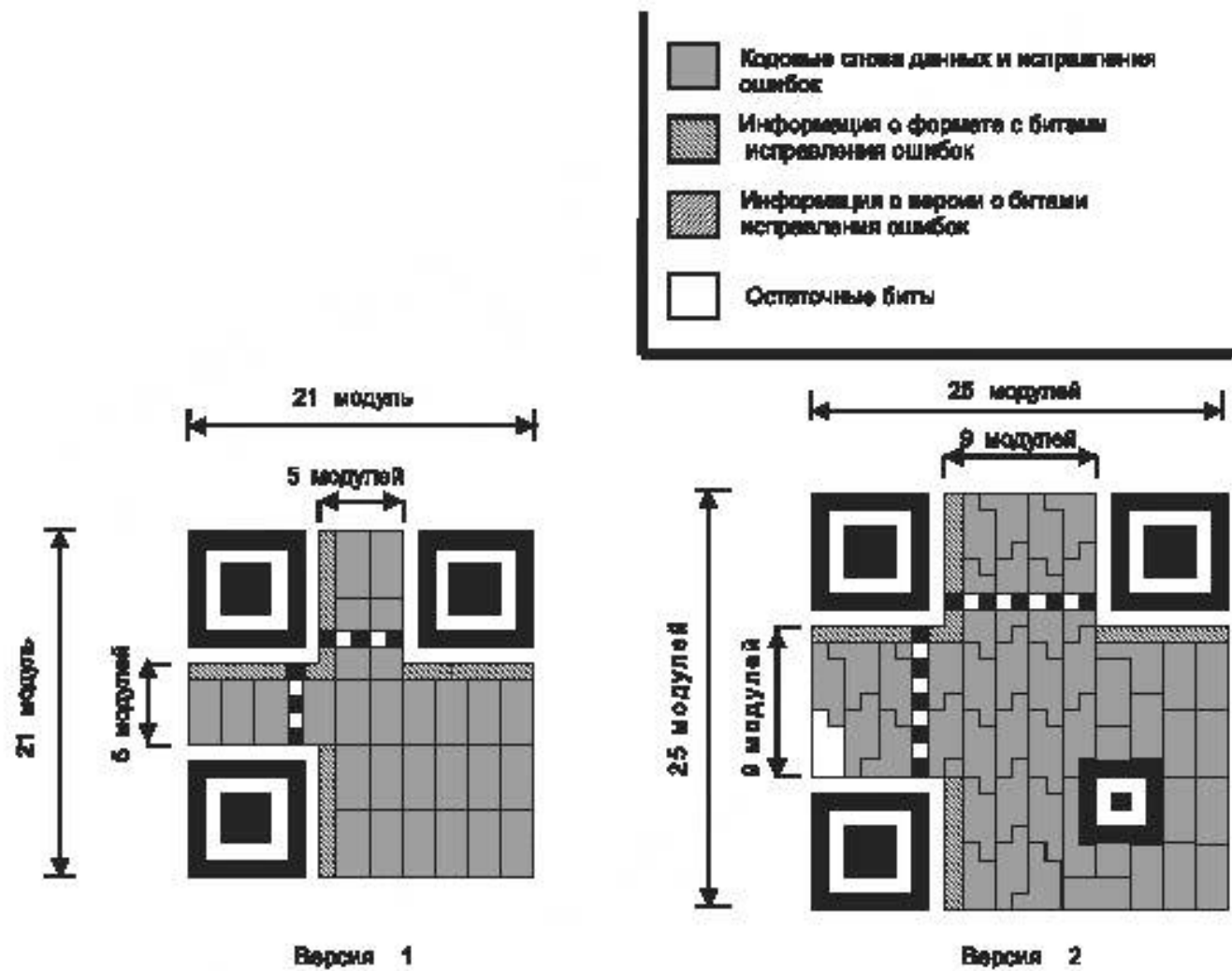
Рисунок 5 — Символы версий 1 и 2
