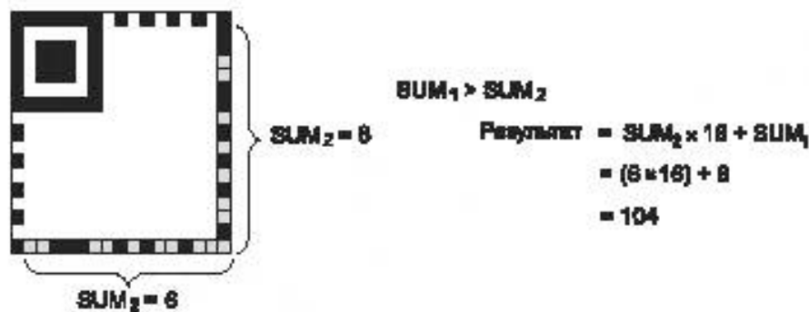
Рисунок 24 – Оценка результата маскирования для Micro QR Code
