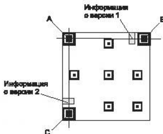
Рисунок 33 – Шаблоны поиска и информация о версии
