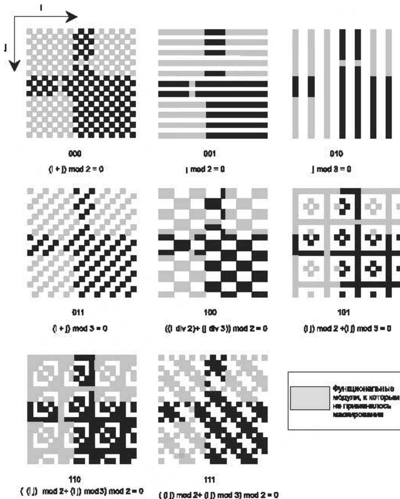
Рисунок 21 – Шаблоны маски данных для символа версии 1
