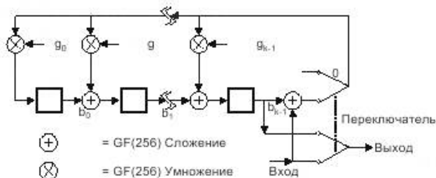
Рисунок 14 — Схема кодирования кодовых слов исправления ошибок
