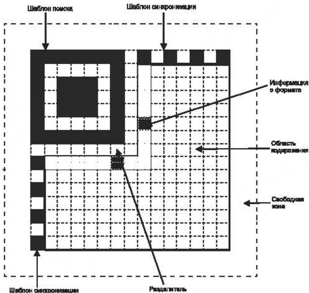
Рисунок 4 — Структура символа Micro QR Code версии M3
