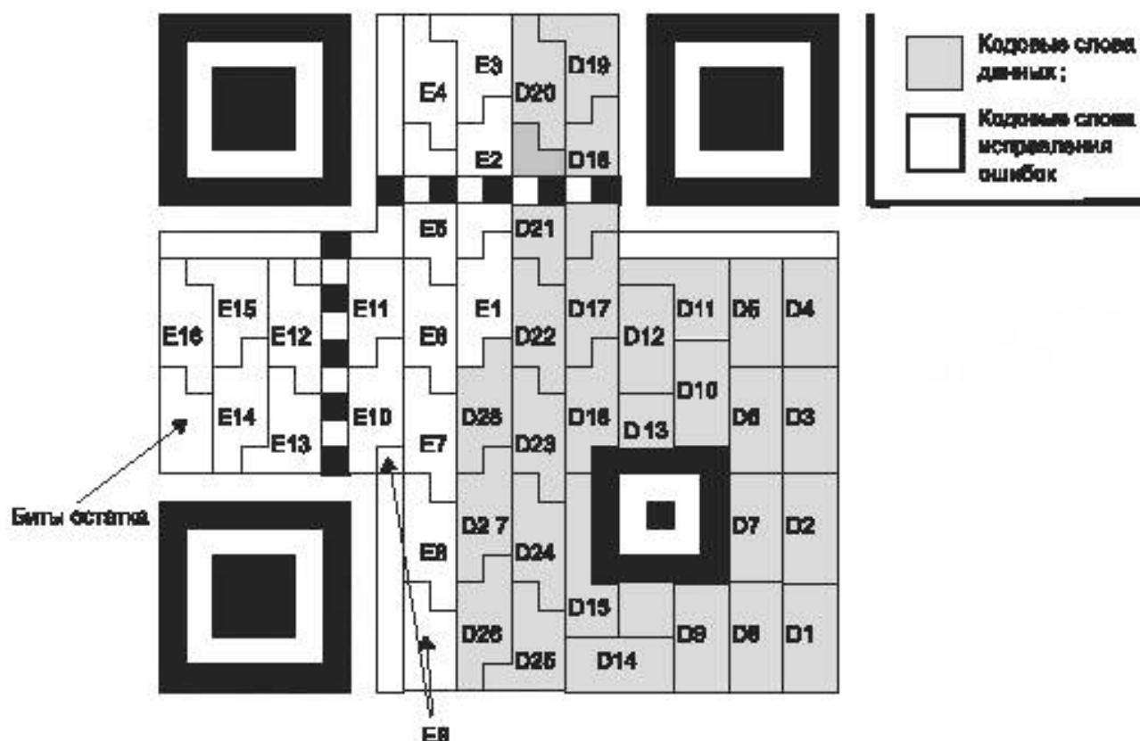
Рисунок 19 – Размещение знаков символа версии 2-M
