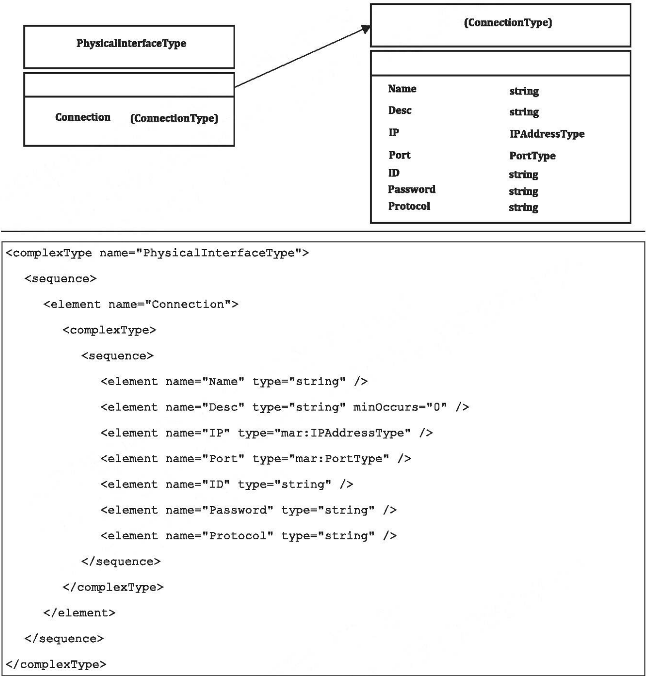
Рисунок 43 — Тип физического интерфейса
