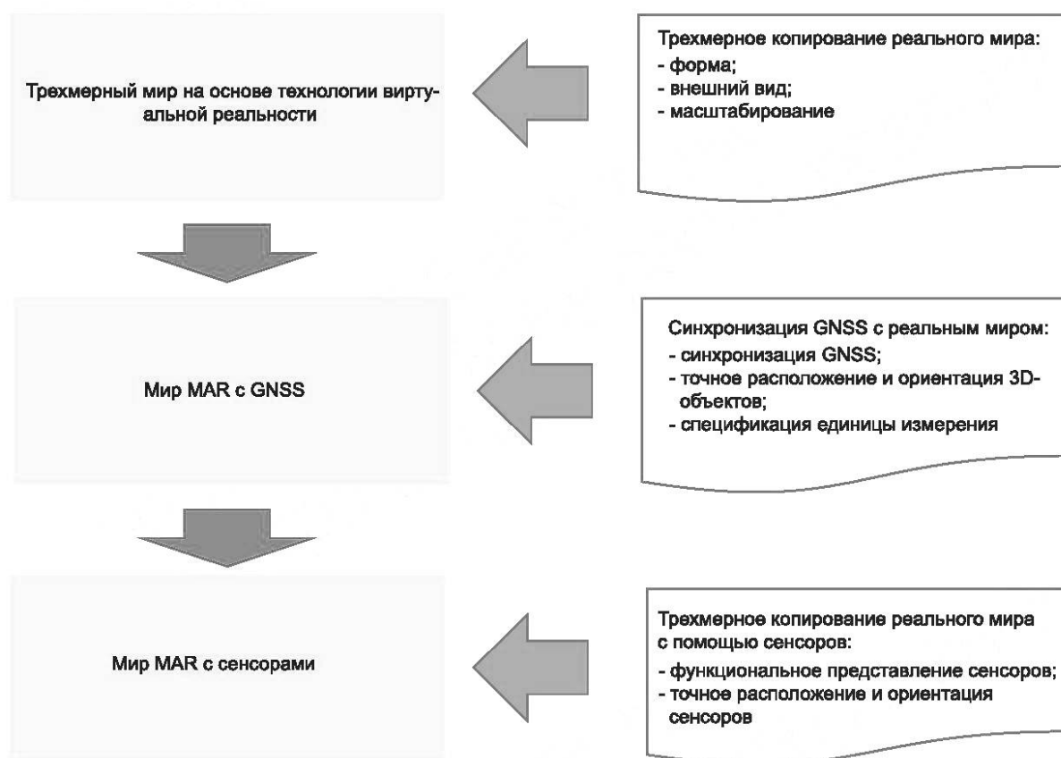
Рисунок 19 — Создание мира сенсоров MAR
