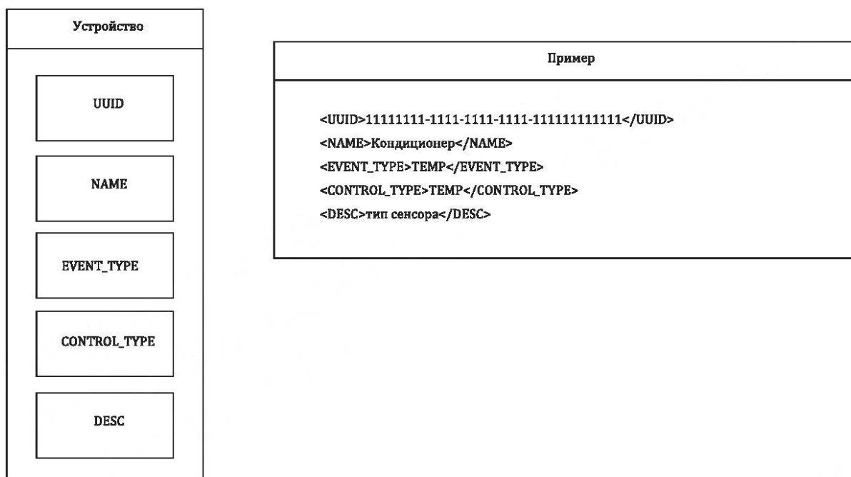
Рисунок 25 — Физические свойства физического сенсора
