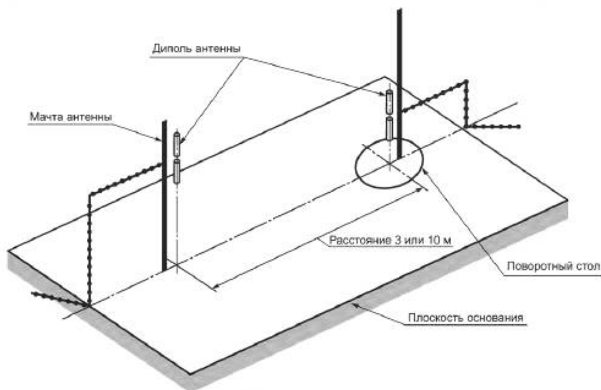
Рисунок А.3 — Типичная открытая испытательная площадка
