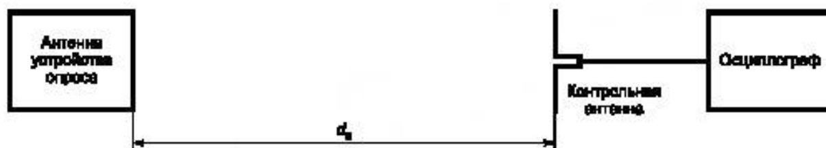
Рисунок 1 — Установка для испытаний модуляции устройства опроса
