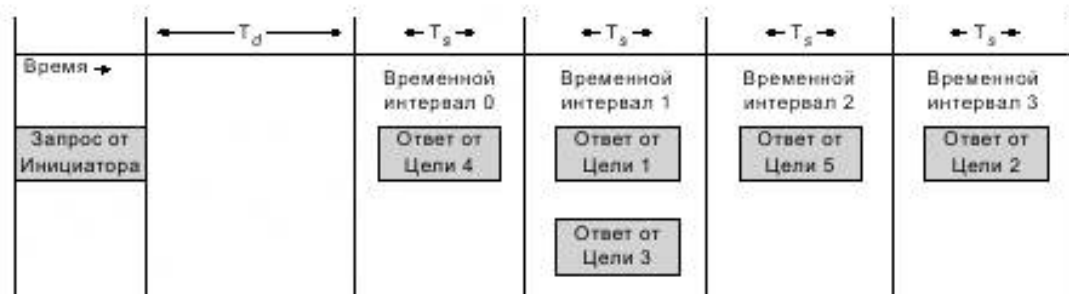
Рисунок 9 — Обнаружение единственного устройства по временным интервалам
