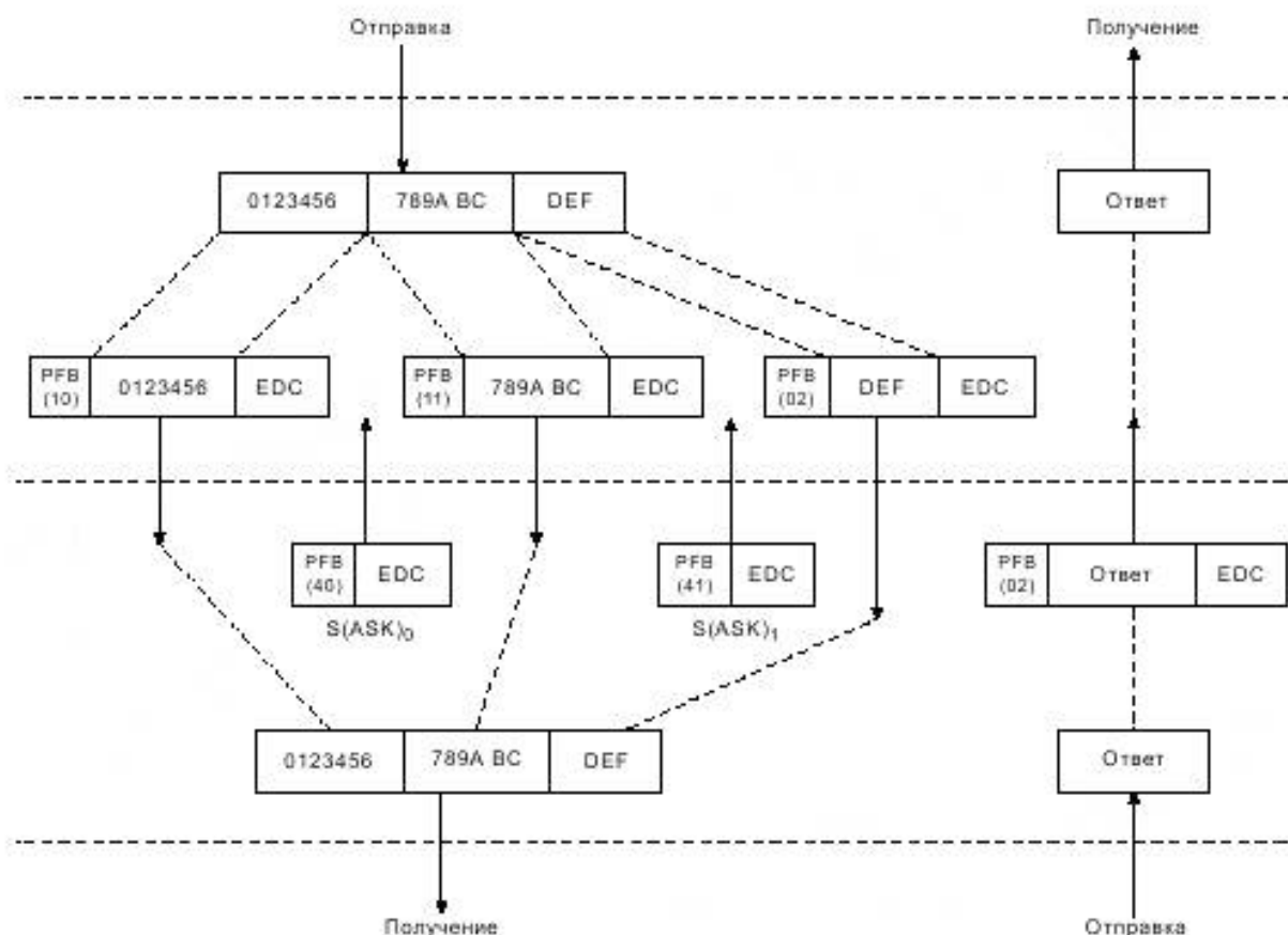
Рисунок 36 — Больше информации (формирование цепочки)
