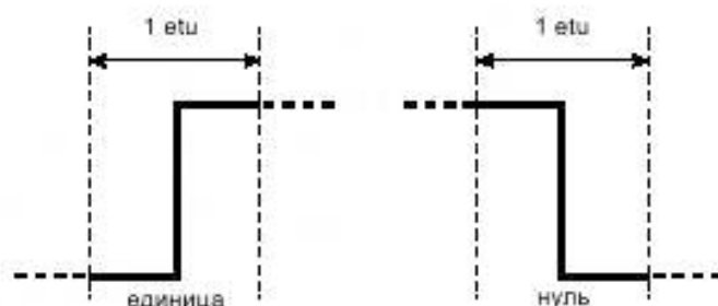
Рисунок 2 — Манчестерское двоичное кодирование (обратная амплитуда)
