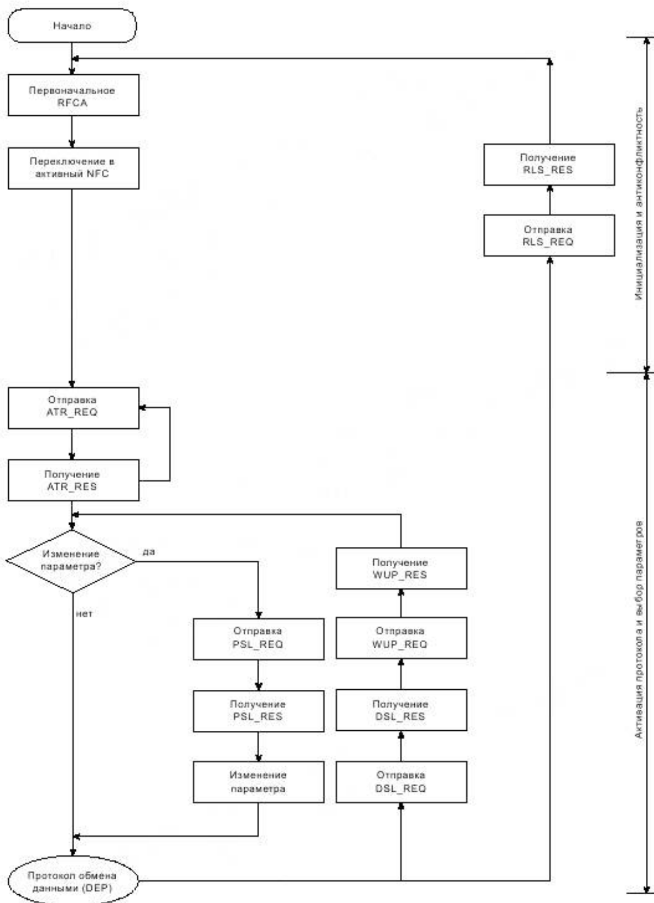
Рисунок 15 — Протокол активации в активном режиме связи
