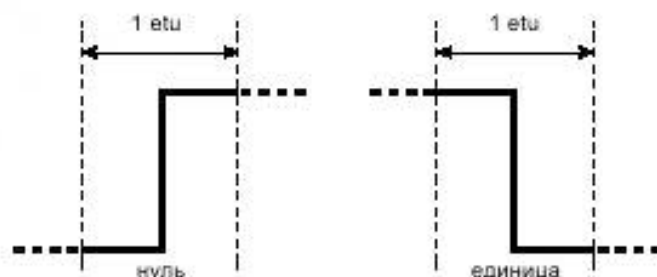
Рисунок 1 — Манчестерское двоичное кодирование (прямая амплитуда)
