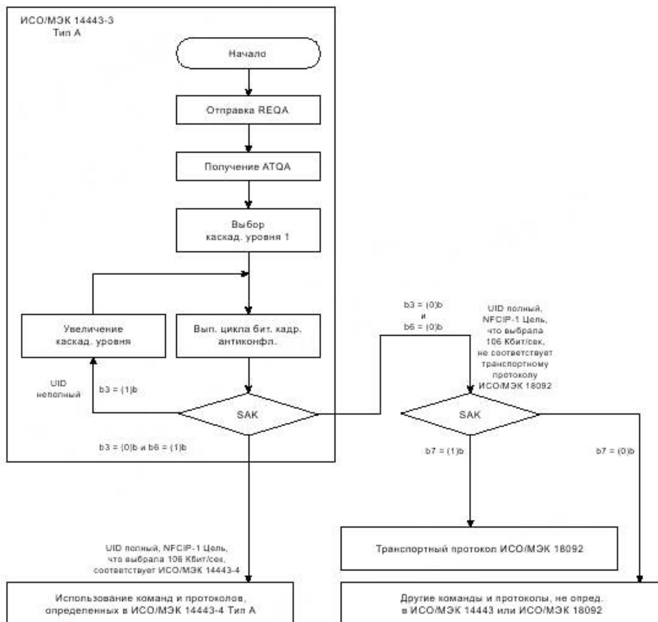
Рисунок В.1 — Комбинация SAK
