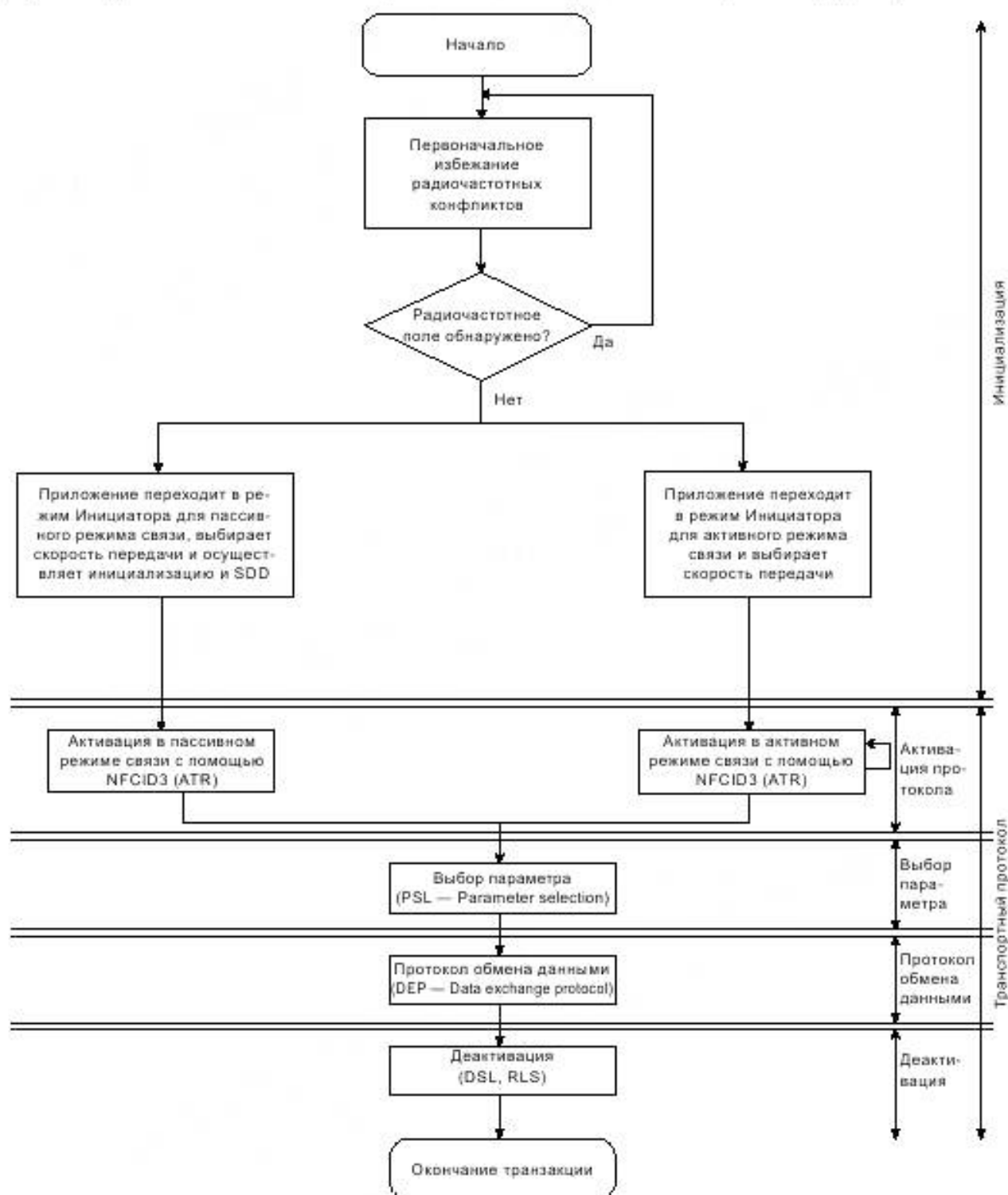
Рисунок 3 — Общий ход инициализации и обнаружения единственного устройства
