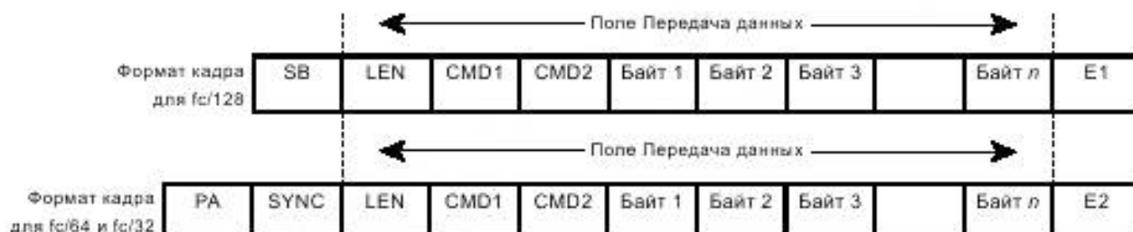
Рисунок 13 — Формат кадра передачи данных
