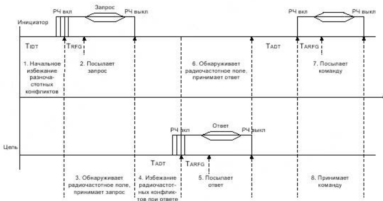
Рисунок 12 — Ход выполнения инициализации в активном режиме связи
