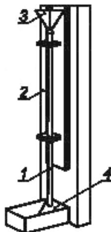
1 — стеклянная трубка; 2 — штатив; 3 — конусообразная воронка; 4 — ящик
