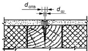
Рисунок Г.3 — Крепление внутренней обшивки шурупами
