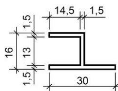
Рисунок В.1 — Профиль ПС 885-265
