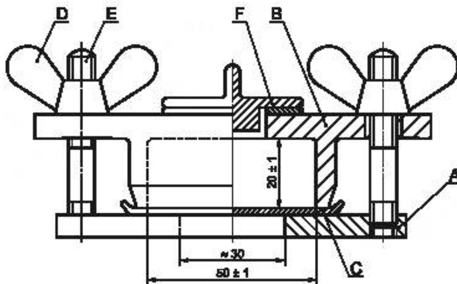
Рисунок 1 — Аппарат для испытания только одной поверхности образца
