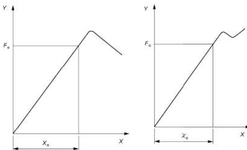
Рисунок 1 — Пример кривой «нагрузка — перемещение» (метод В)
