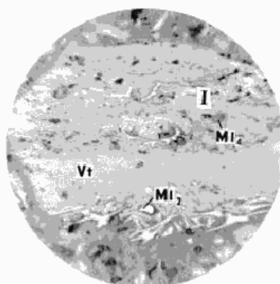
Сросток микролитотипа 2-й группы (V + F) + + кварц (MI 1 ) + пирит (MI 2 )
