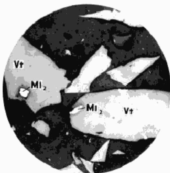
Сростки микролитотипов 1-й группы (V) + + пирит (MI 2 )
