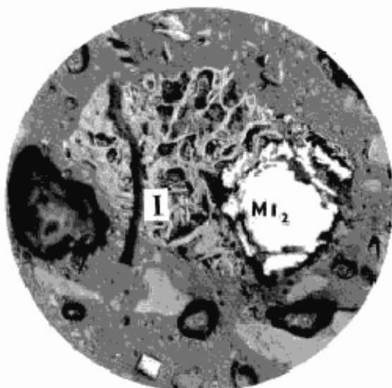
Сросток микролитотипа 3-й группы ( F ) + + пирит ( MI_2 )
