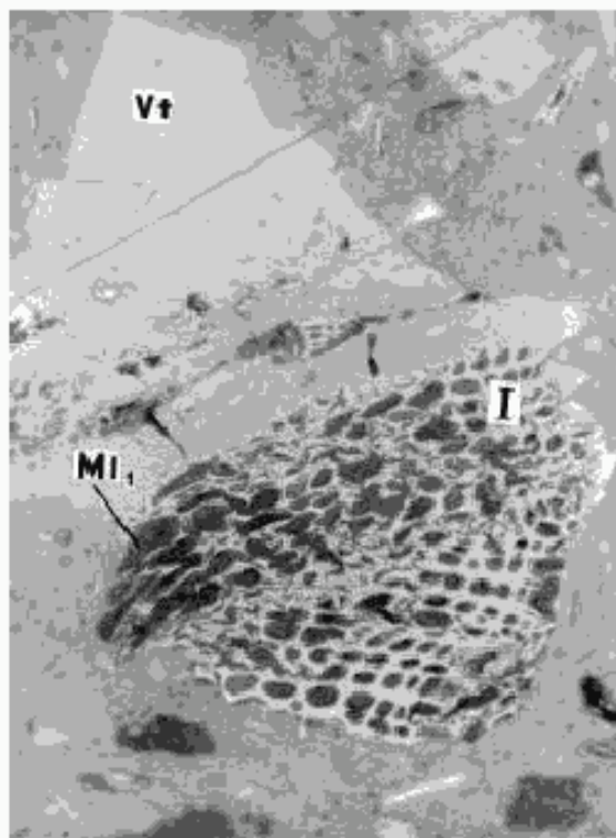
Сросток микролитотипа 2-й группы (V + F) + аргиллит (Ml 1 ) Черт. 6
