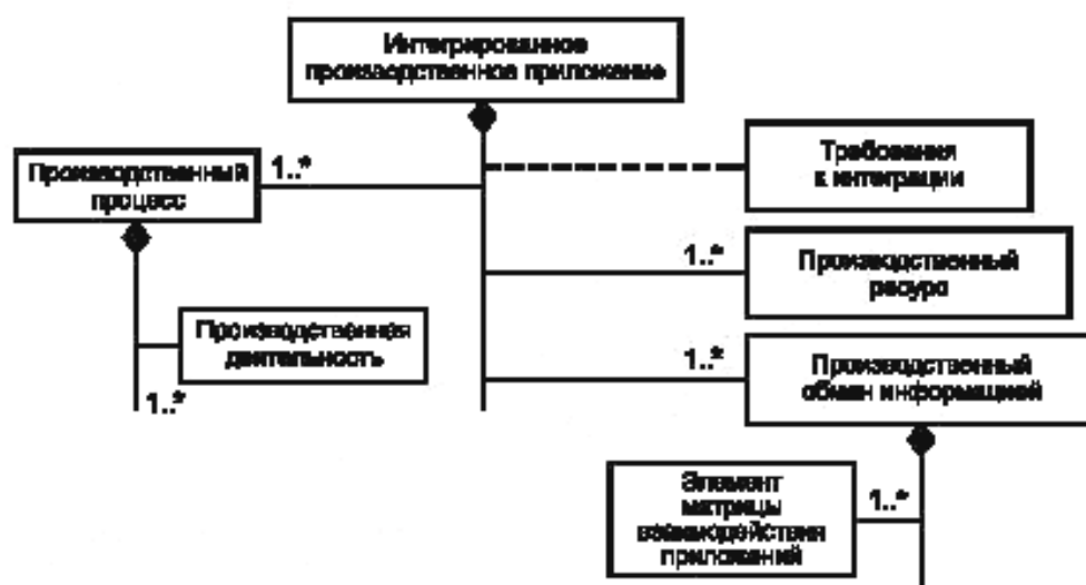
Рисунок 6 — Диаграмма соотношений интеграции приложений (AIRD)
