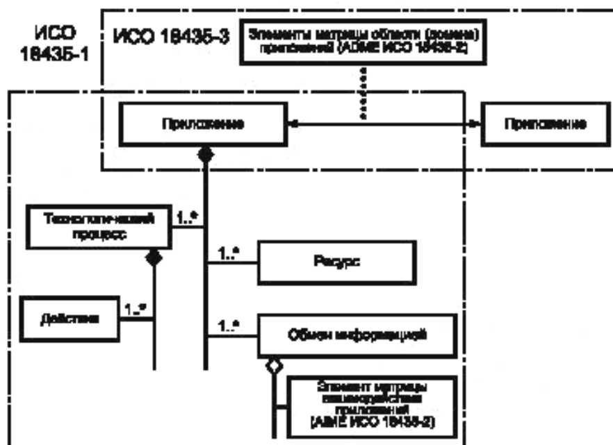
Рисунок 3 — Соотношения внутри комплекса международных стандартов ИСО 18435
