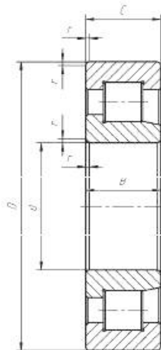
Рисунок 2 – Конструктивное исполнение 42000 с однобортиковым внутренним кольцом
