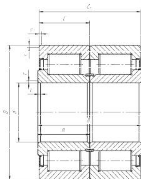
Рисунок 9 – Конструктивное исполнение 882000 – Сдвоенный подшипник с защитными шайбами/уплотнениями
