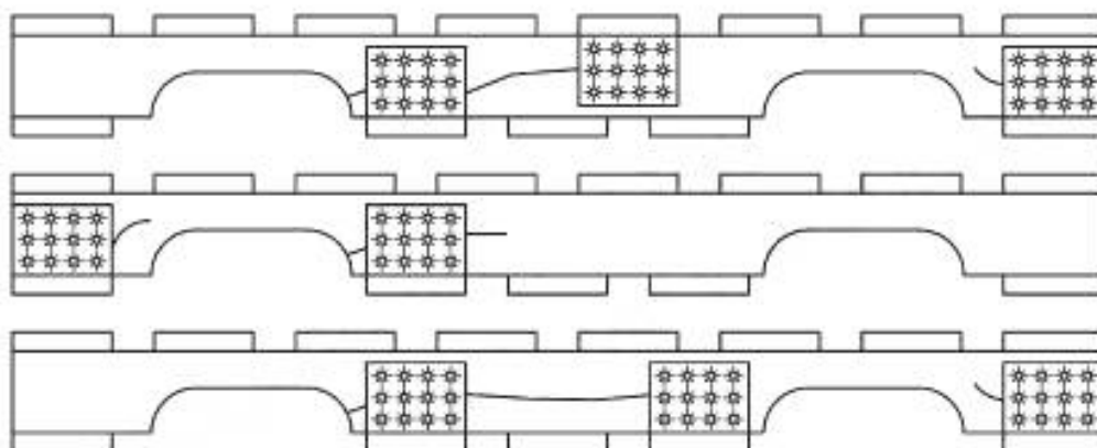
Рисунок Е.2 — Прикрепление соединительных металлических пластин
