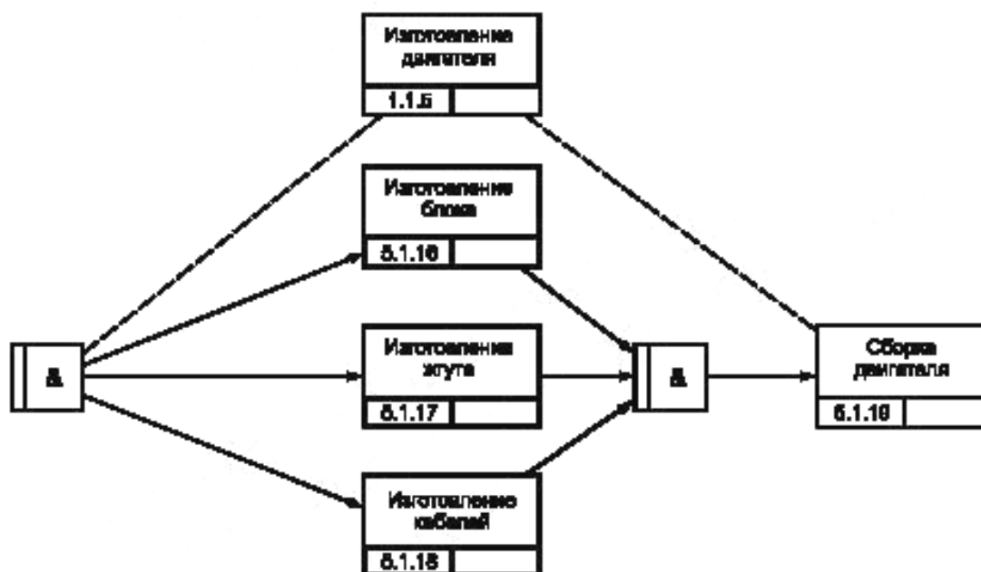
Рисунок В.2 — Процесс изготовления двигателя изделия GT-350 [4]
