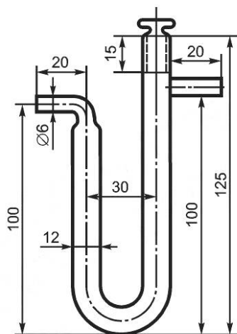
Рисунок 4 — U-образная трубка
