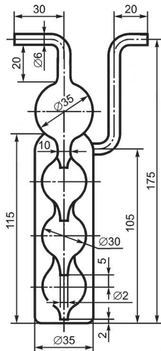
Рисунок 6 — Поглощительная склянка
