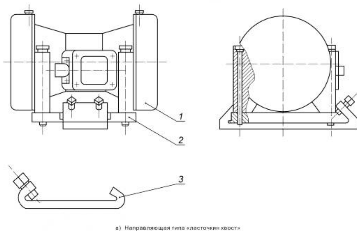
Рисунок А.6 — Конструкции быстросъемных устройств для электрических внешних вибраторов съемного типа
