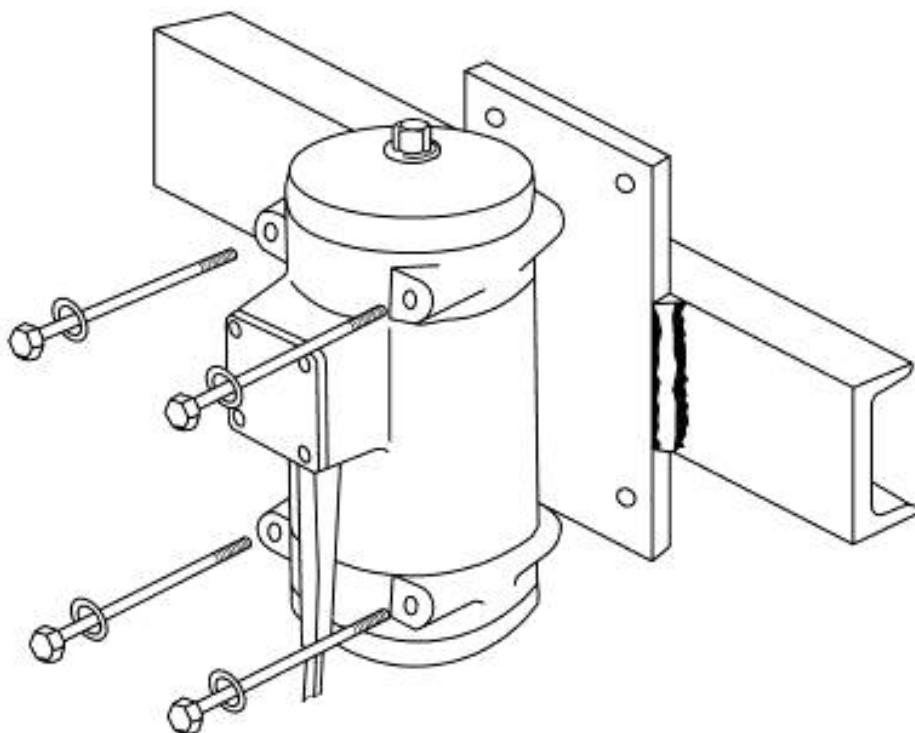
Рисунок А.5 — Крепления электрического внешнего вибратора фиксированного типа
