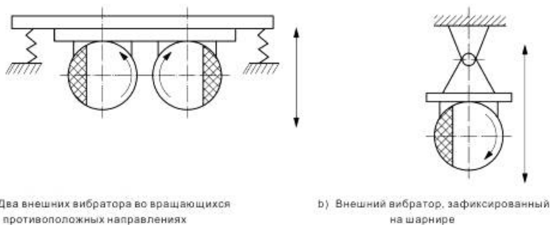
Рисунок А.10 — Принцип работы внешних вибраторов направленного действия
