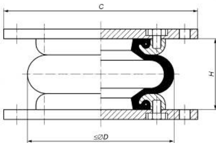
Рисунок В.4 — Основные размеры пневматической рессоры
