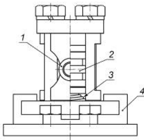
1 — цилиндр; 2 — поршень; 3 — пружина; 4 — станина
