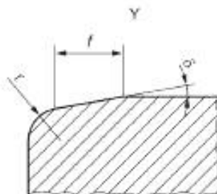
Рисунок 9 — Закругленная кромка (выносной элемент Y рисунка 6)
