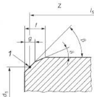
Рисунок 10 — Наружная кромка с фиксирующей фаской для круглого стопорного кольца
