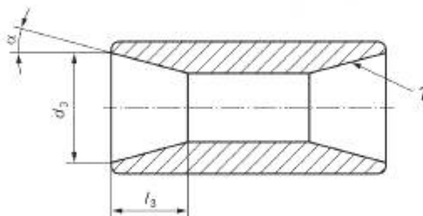
Рисунок 4 – Палец с холодноштампованной концевой перегородкой
