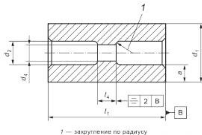
Рисунок 17 — Размеры центральной перегородки
