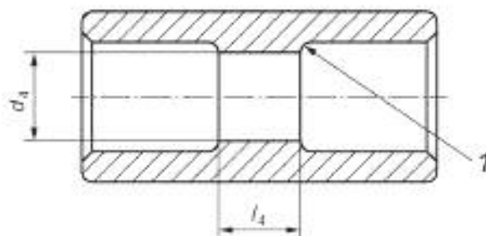
Рисунок 2 – Выносной элемент W рисунка 1
