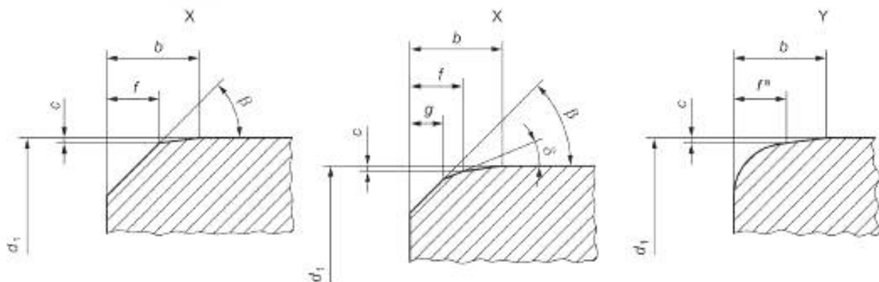
а) Скошенная кромка и уклон
