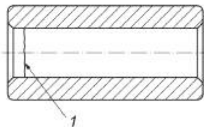
Рисунок 3 – Палец с холодноштампованной центральной перегородкой
