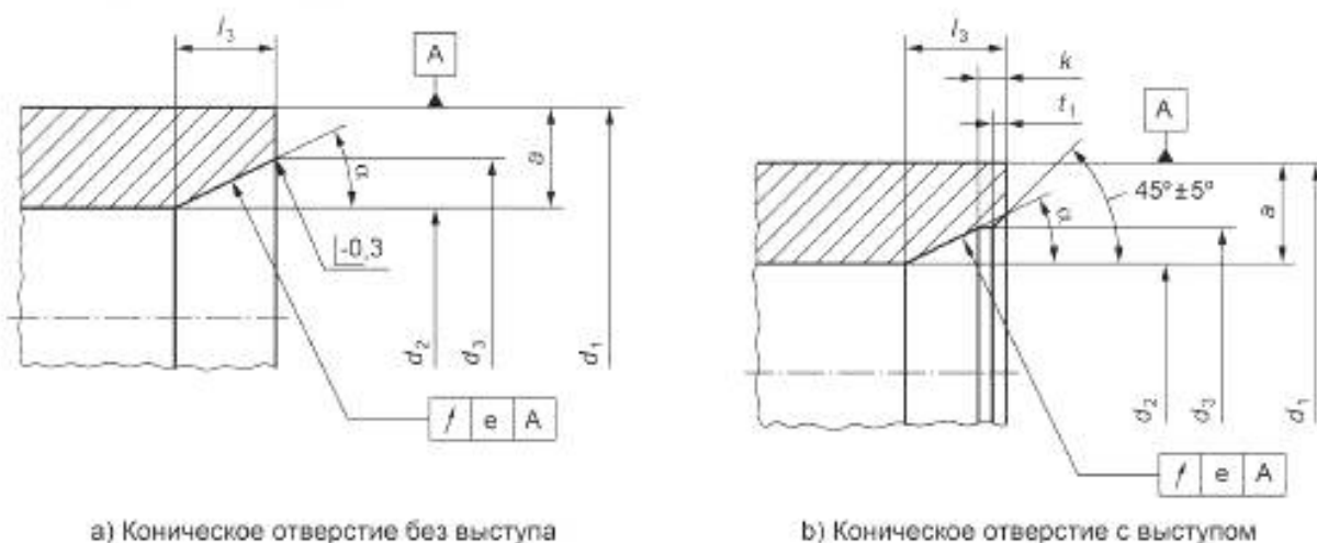
Рисунок 16 — Варианты конического отверстия
