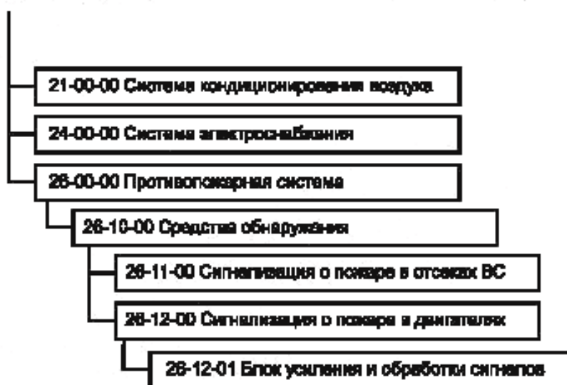
Рисунок 2 — Использование СНК для идентификации СЧ ВС
