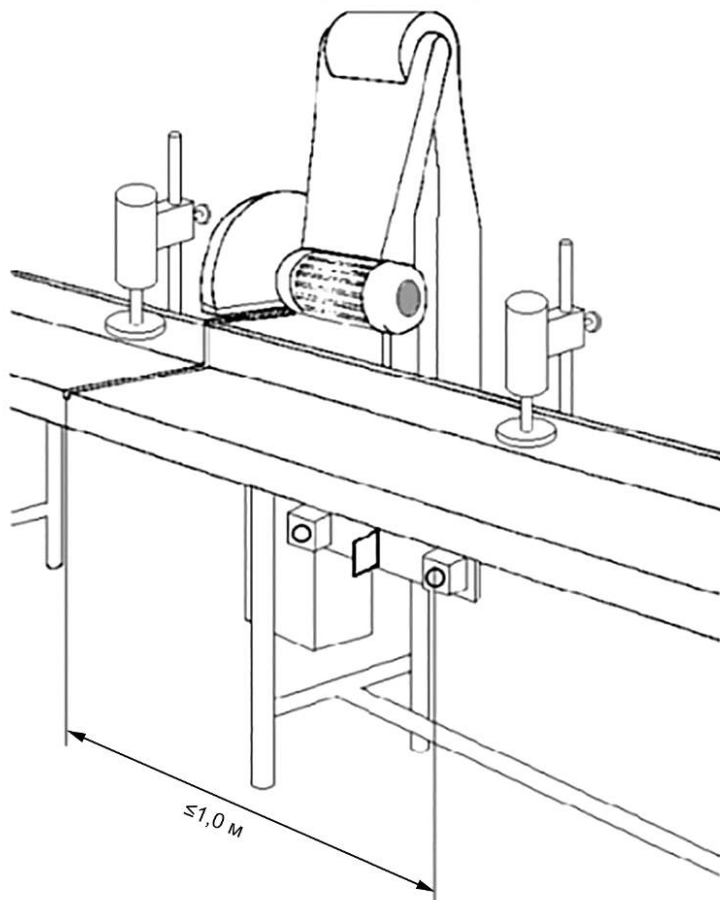
Рисунок 2 — Расположение двухручного устройства управления на полуавтоматических станках
