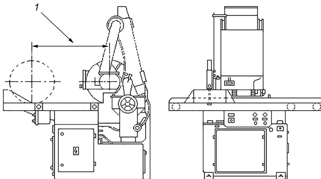
1 — ход дисковой пилы
