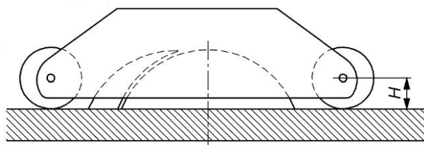
Рисунок 19 — Размеры скоса у передней кромки защитного ограждения дисковой пилы, закрепленного на столе станка отдельно от расклинивающего ножа
