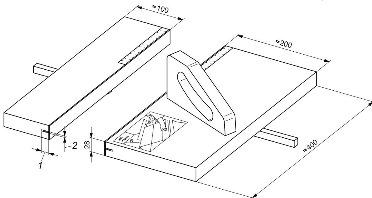
Рисунок 26 — Пример второго безопасного устройства для распиливания
