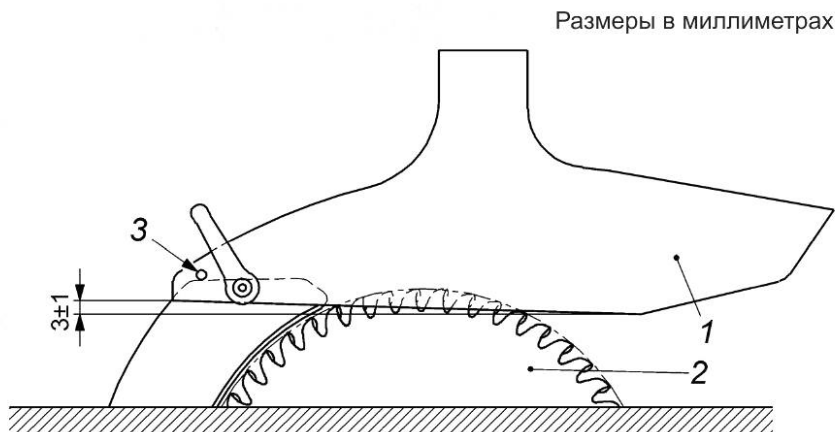
1 — защитное ограждение дисковой пилы в верхнем положении; 2 — дисковая пила отрегулирована на максимальную глубину пропила; 3 — концевой упор
