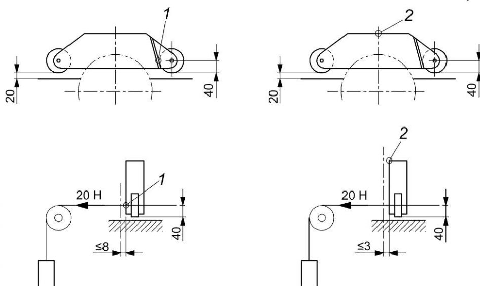
Рисунок Е.2 — Испытание на устойчивость для защитных ограждений дисковой пилы с направляющими роликами, устанавливаемых отдельно от раскливающего ножа
