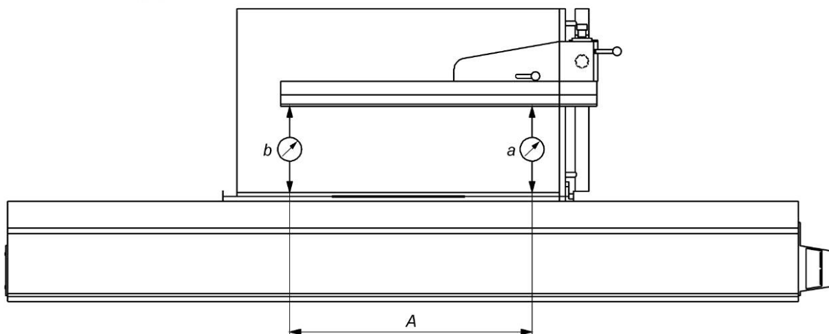
A — измеряемое расстояние; a — точка измерения для e_j ; b — точка измерения для e_k
