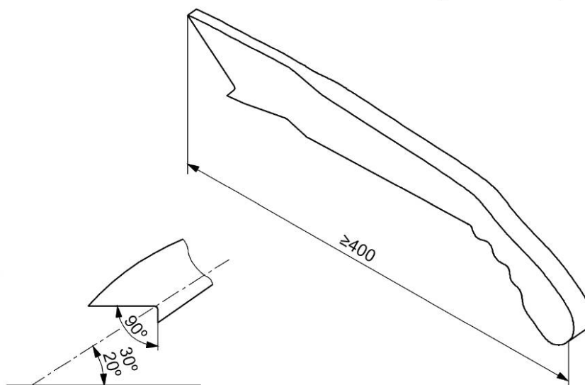
Рисунок 24 — Примеры толкателя
