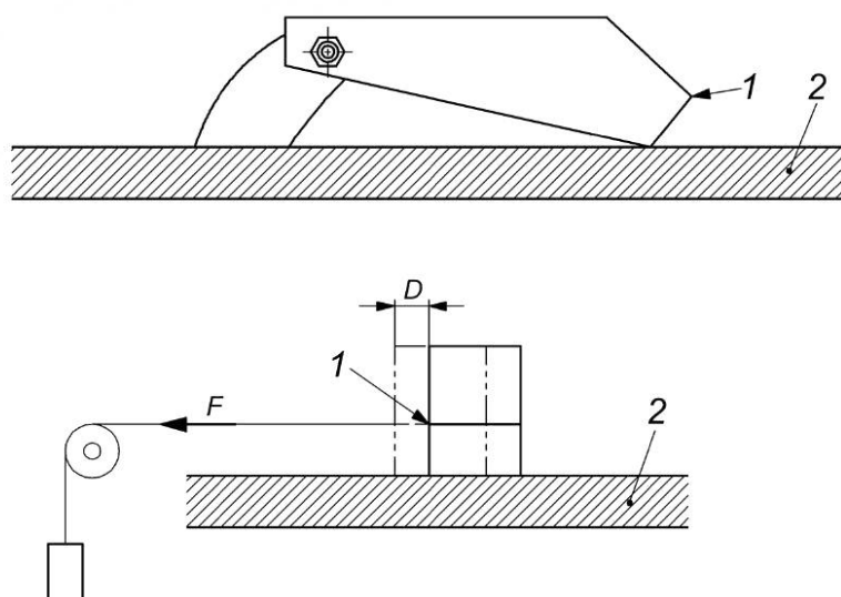
Рисунок Е.3 — Испытание на устойчивость для защитных ограждений дисковой пилы, устанавливаемых на раскливающем ноже с направляющими роликами
