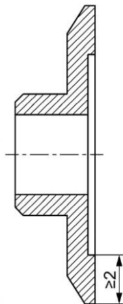
Рисунок 3 — Деталь фланца пилы (зажимная поверхность)
