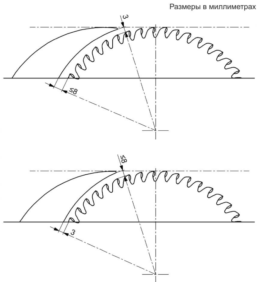
Рисунок 8 — Расположение зазоров для расклинивающего ножа
