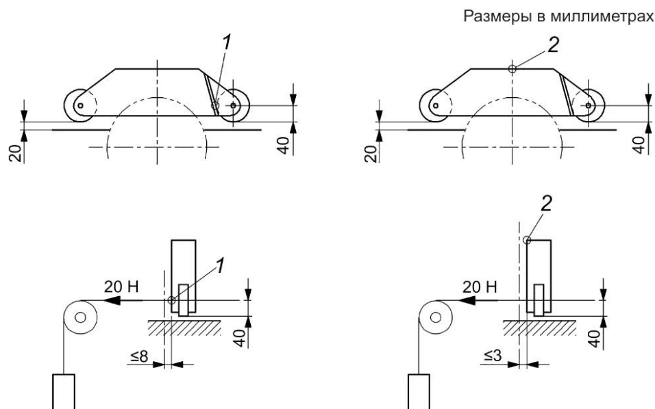
Рисунок G.2 — Испытание на устойчивость для защитных ограждений дисковой пилы с направляющими роликами, устанавливаемых отдельно от расклинивающего ножа
