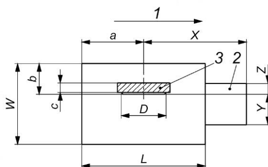
Рисунок F.1 — Размеры стола станка, удлинителя стола и вставки стола станков
