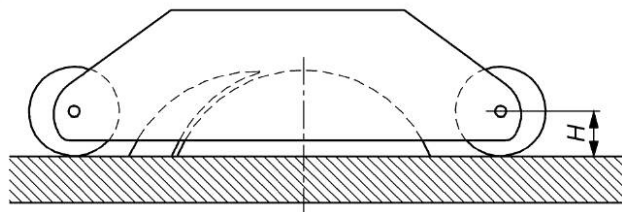
Рисунок 22 — Размеры роликов передней кромки защитного ограждения дисковой пилы, закрепленного на столе станка отдельно от расклинивающего ножа
