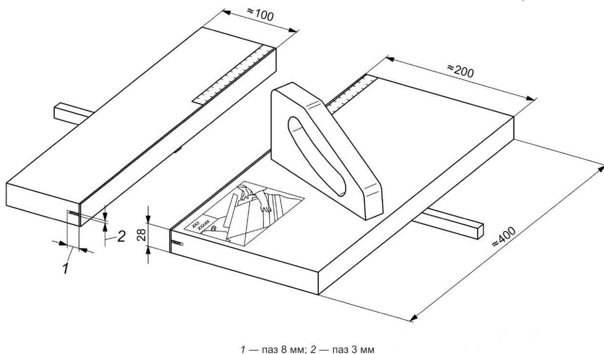
Рисунок 31 — Пример второго безопасного устройства для распиливания
