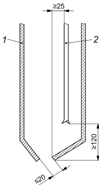
1 — защитное ограждение дисковой пилы под столом станка; 2 — дисковая пила
