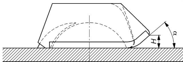
Рисунок 21 — Размеры скоса передней кромки защитного ограждения дисковой пилы, закрепленного на столе станка отдельно от расклинивающего ножа
