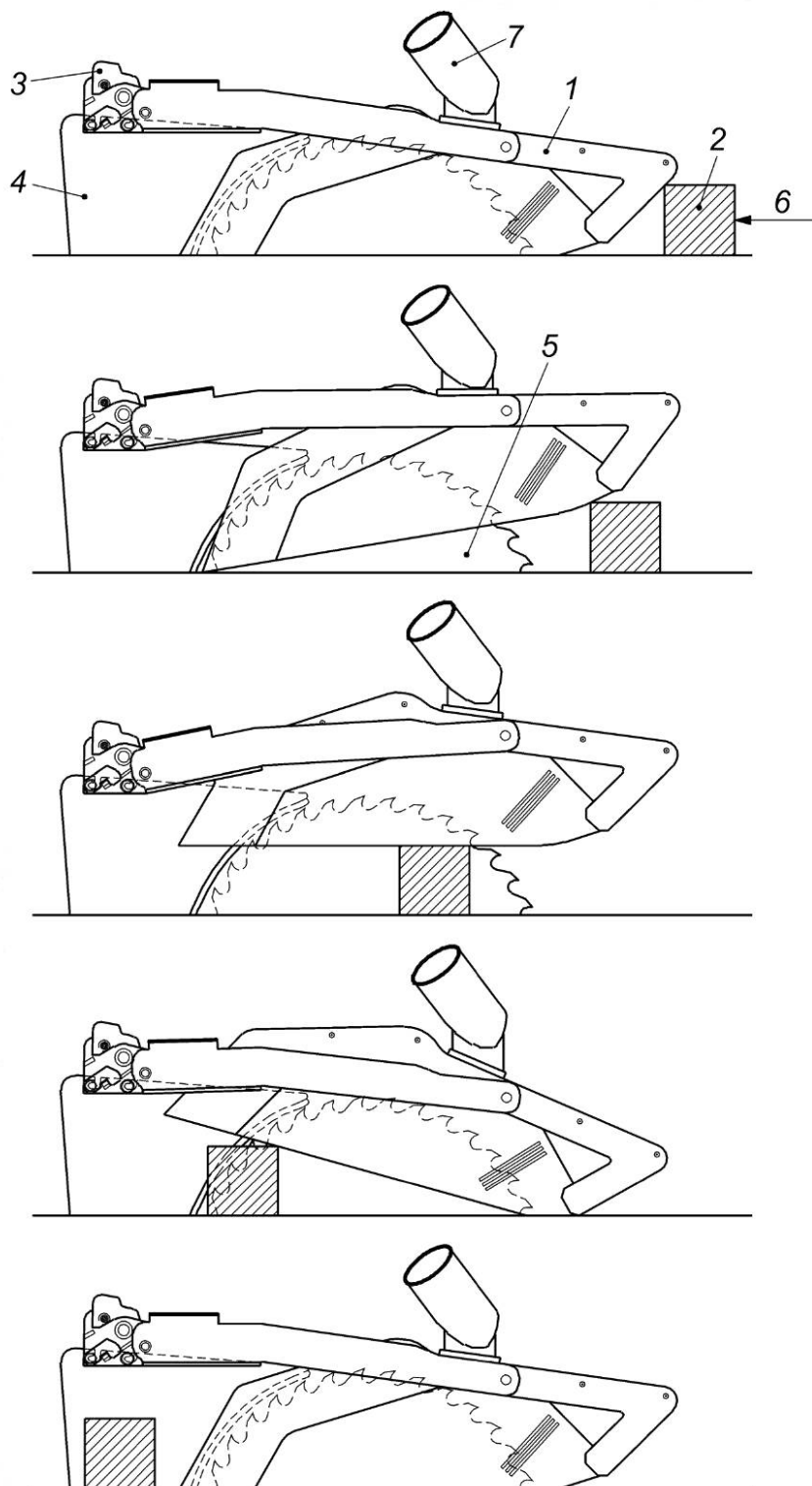
1 — держатель верхнего защитного ограждения; 2 — обрабатываемая заготовка; 3 — крепление верхнего защитного ограждения на расклинивающем ноже; 4 — расклинивающий нож; 5 — дисковая пила; 6 — направление подачи; 7 — вытяжное отверстие
