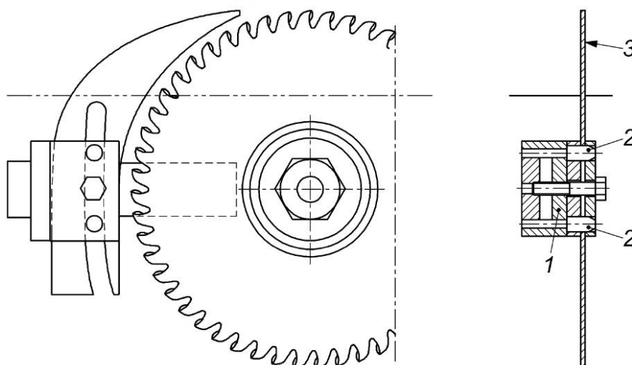
1 — крепление расклинивающего ножа; 2 — направляющие штифты; 3 — расклинивающий нож
