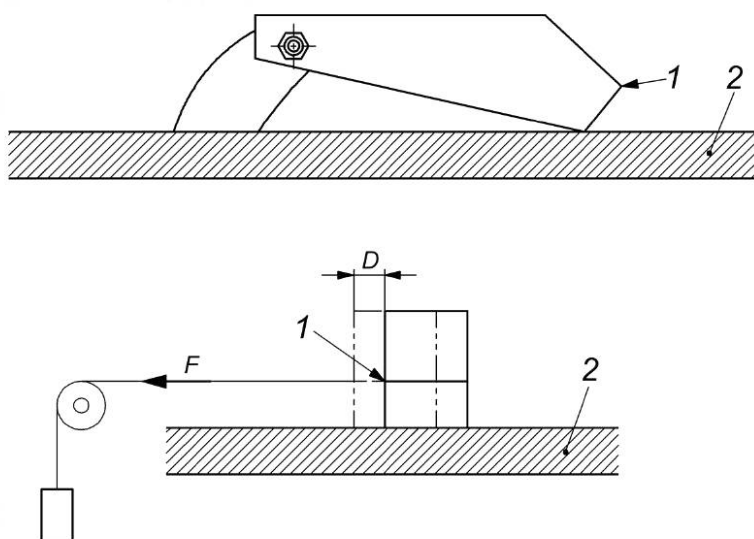
Рисунок G.3 — Испытание на устойчивость для защитных ограждений дисковой пилы, устанавливаемых на расклинивающем ноже с направляющими роликами
