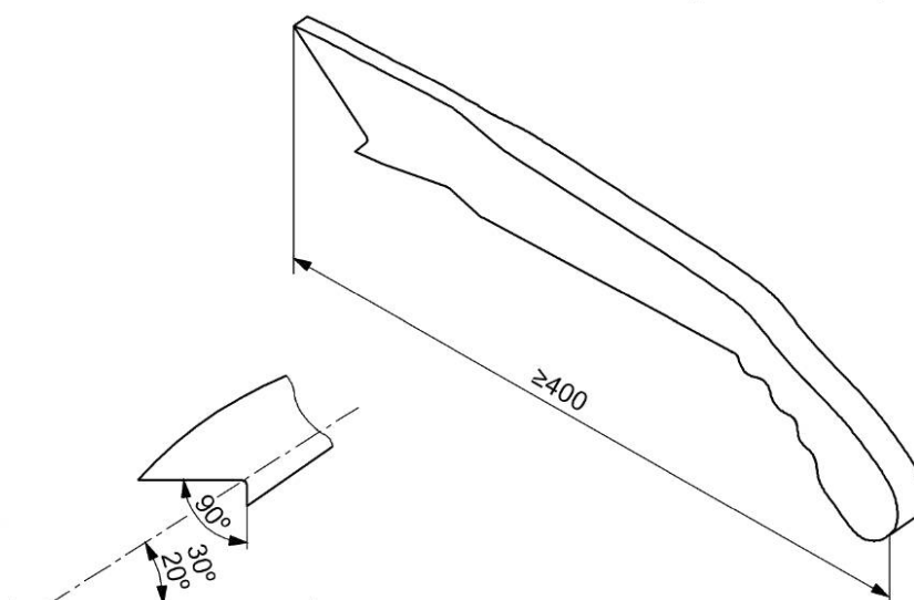
Рисунок 29 — Примеры толкателя
