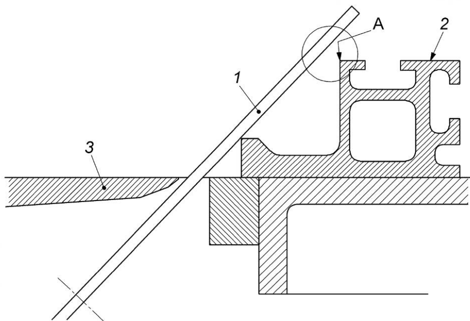
Рисунок 15 — Положение направляющей планки в низком положении
