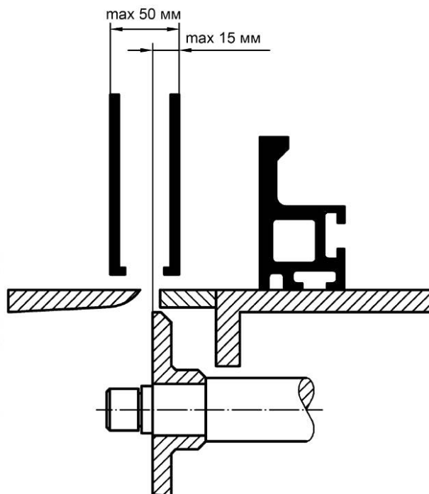
Рисунок 20 — Максимальная ширина защитного ограждения пилы
