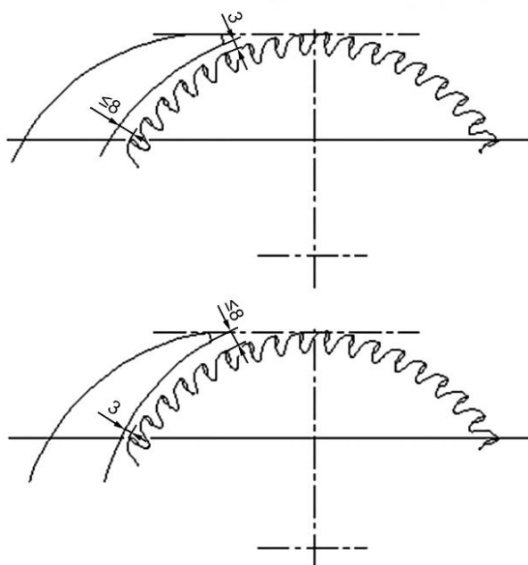
Рисунок 12 — Размеры при установке расклинивающего ножа
