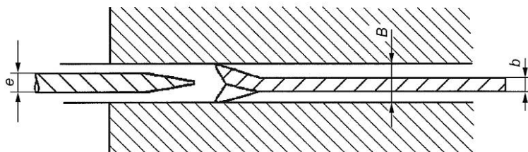
e — толщина расклинивающего ножа; b — толщина пилы; B — ширина пропила
