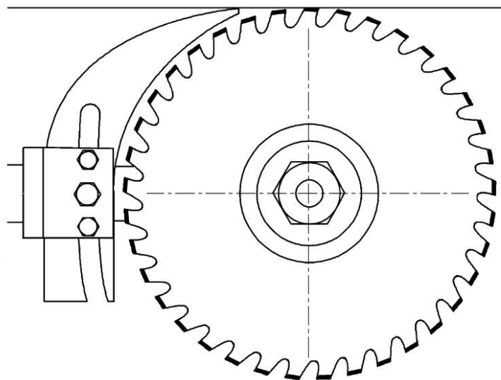
Рисунок 11 — Регулировка высоты расклинивающего ножа
