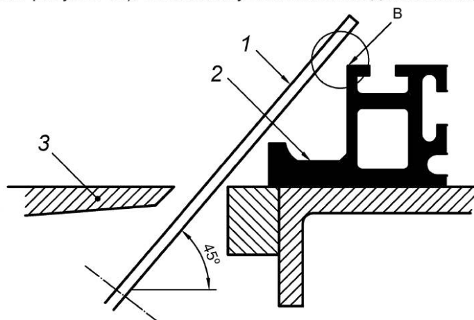
1 — пила; 2 — направляющая в нижней позиции; 3 — стол
