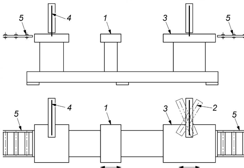
1 — регулируемая центральная опора; 2 — устройство регулировки угла обработки (при наличии); 3 — регулируемое пильное устройство; 4 — дисковая пила; 5 — роликовый конвейер (опция)
