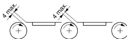
Рисунок 5б) — Конвейер с подающими роликами
