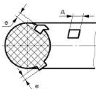
Рисунок 3 — Отклонения — возвышения и углубления поверхности
