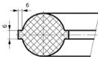
Рисунок 1 — Отклонения — выпрессовка
