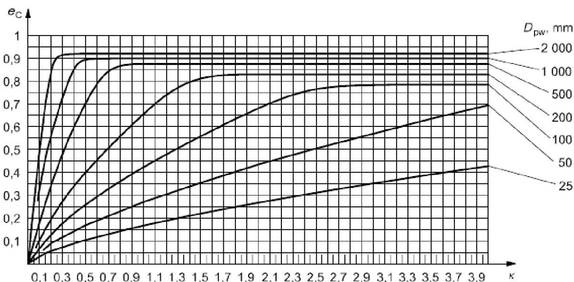
Рисунок А.1 — Коэффициент e_c для циркуляционного масляного смазывания со встроенными фильтрами — \beta_{6(c)} = 200 , код по ISO 4406 -/13/10
