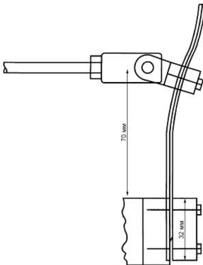
Рисунок 1 — Конфигурация верхнего и нижнего зажимов
