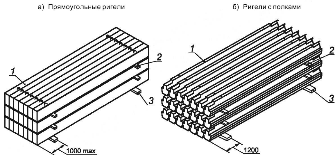
Рисунок 1 — Складирование ригелей
