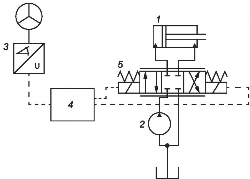
1 — поворотный гидроцилиндр; 2 — насос; 3 — датчик рулевого управления; 4 — ECU; 5 — клапан рулевого управления Рисунок А.1 — Схема электрогидравлического рулевого управления категории В
