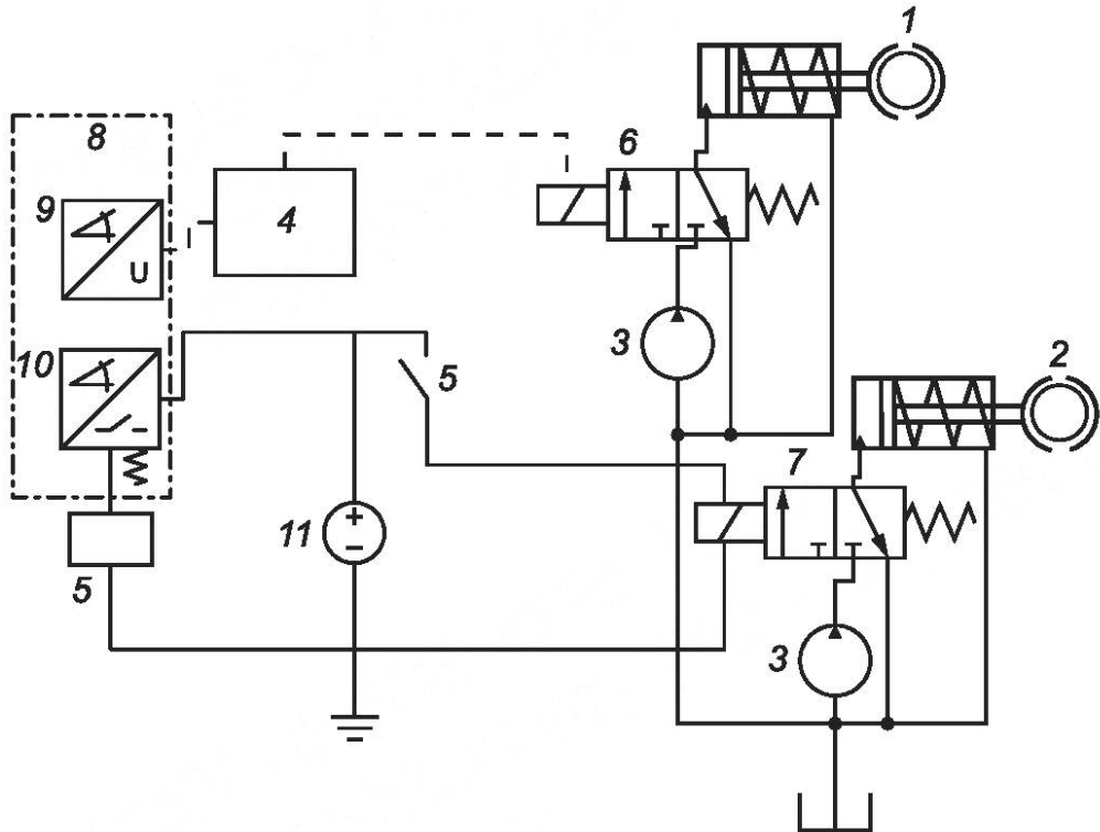
1 — основной тормозной цилиндр; 2 — дополнительный тормозной цилиндр; 3 — насос; 4 — ECU; 5 — реле тормоза; 6 — электромагнитный клапан основной тормозной системы; 7 — электромагнитный клапан дополнительной тормозной системы; 8 — педаль тормоза; 9 — датчик педали; 10 — концевой выключатель конца хода педали; 11 — аккумуляторная батарея
