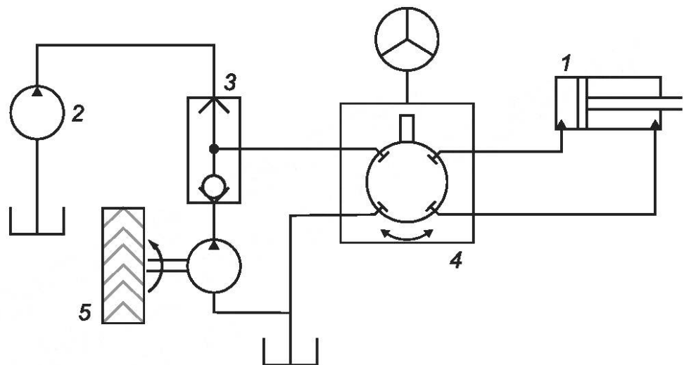
1 — гидроцилиндр рулевого управления; 2 — насос; 3 — челночный клапан; 4 — планетарный клапан; 5 — насос с приводом от ходового колеса
