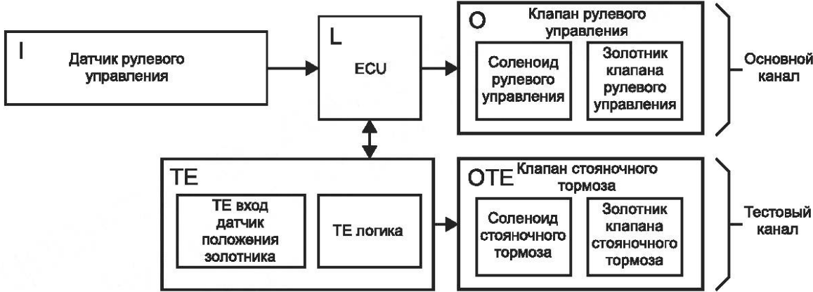
Рисунок А.8 — Логическая схема электрогидравлического рулевого управления с автоматическим стояночным тормозом, категория 2
