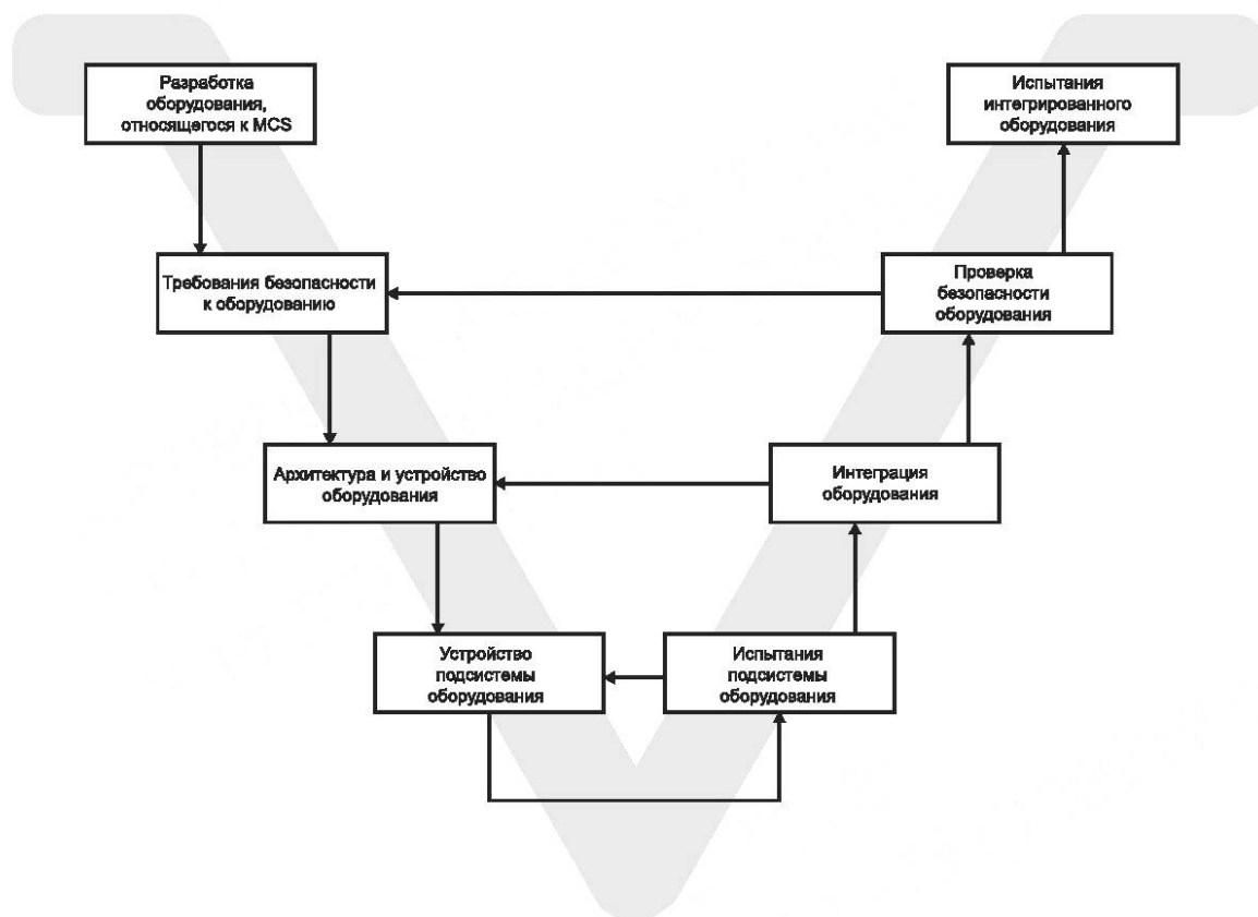
Рисунок 1 — V-модель разработки оборудования
