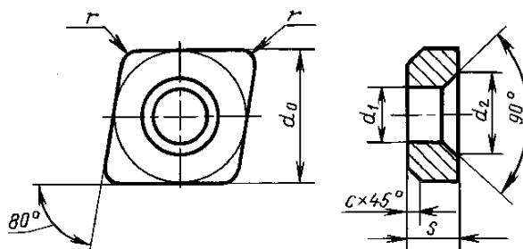
Размеры, мм
