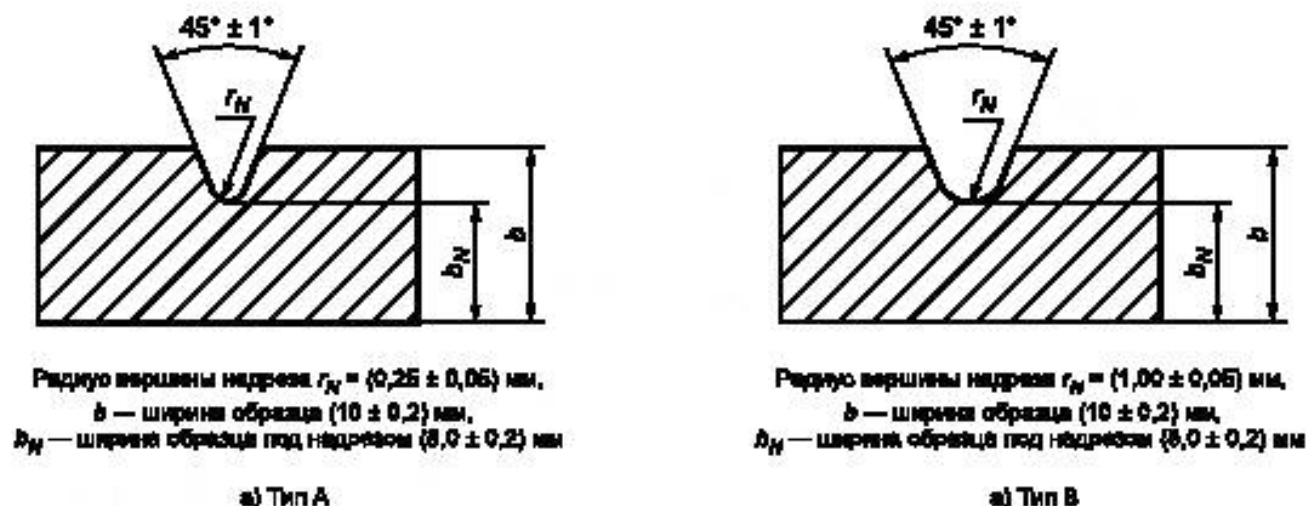
Рисунок 3 — Типы надрезов
