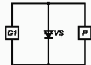
G1 — генератор отпирающих импульсов; P — измеритель временных интервалов; VS — испытуемый тиристор
