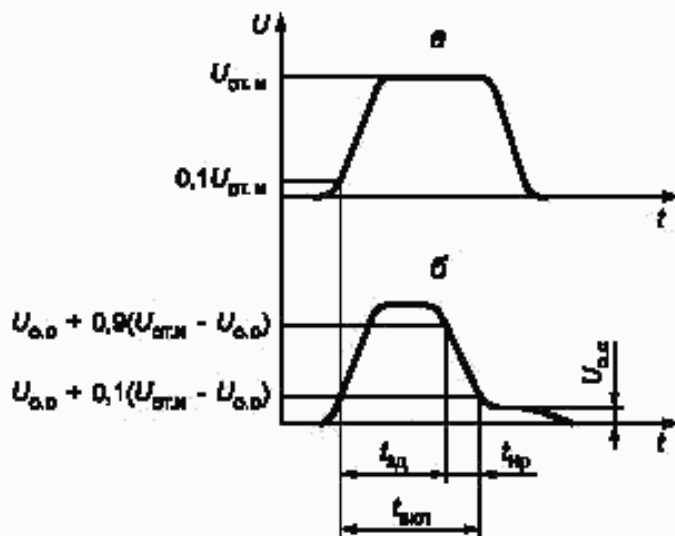
a — форма напряжения на выходе генератора GI при отсутствии испытуемого тиристора; b — форма напряжения на испытуемом тиристоре; U_{о.в} — постоянное напряжение в открытом состоянии тиристора; U_{от.м} — импульсное отпирающее напряжение тиристора
