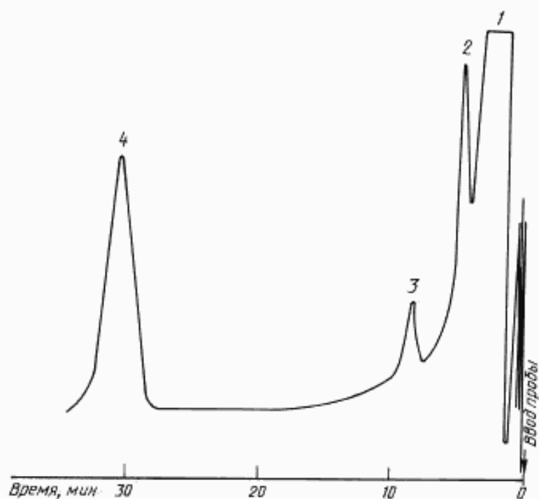
1 — 1,2-дихлорэтан; 2 — 1,1,2-трихлорэтан; 3 — додекан; 4 — 1,1,2,2-тетрахлорэтан
