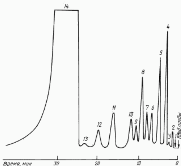
1 — этилен; 2 — винилхлористый; 3 — этил хлористый; 4 — винилиденхлорид; 5 — аллил хлористый; 6 — транс -1,2-дихлорэтилен; 7 — четыреххлористый углерод + 1,1-дихлорэтан; 8 — метилацетилкетон; 9 — метилен хлористый; 10 — бензол; 11 — трихлорэтилен; 12 — хлороформ + перхлорэтилен; 13 — 1,2-дихлорпропан; 14 — 1,2-дихлорэтан
