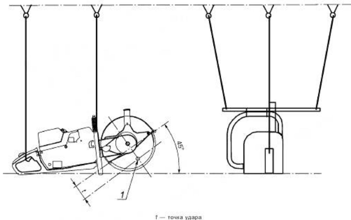
Рисунок А.1 — Испытательный стенд для отрезного диска. Испытание на разрушение
