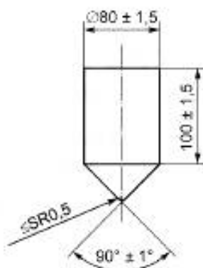
Рисунок 7 — Испытательный конус
