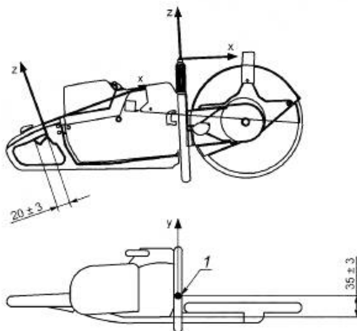
Рисунок С.1 — Расположение акселерометра
