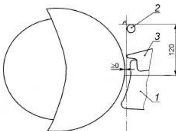
Рисунок 6 — Защита от контакта с горячими частями
