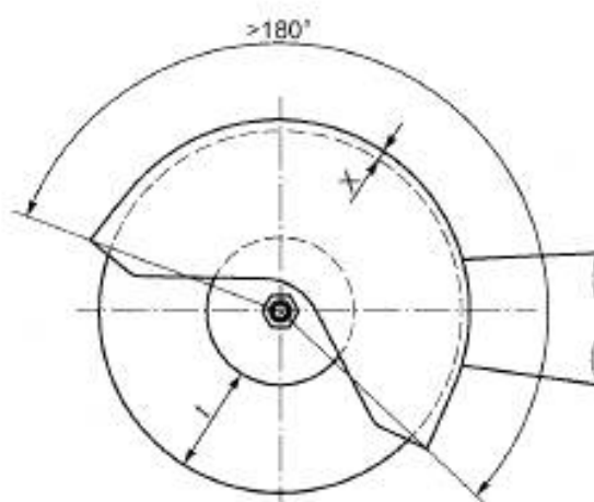
t — максимальная глубина резания; X — радиальный зазор
