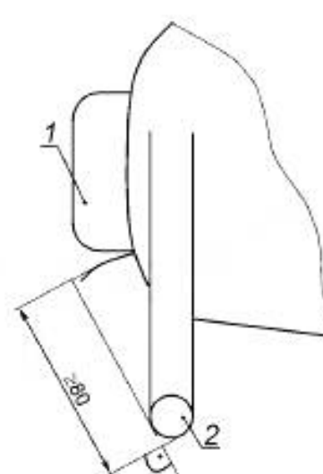
1 — глушитель; 2 — передняя рукоятка
