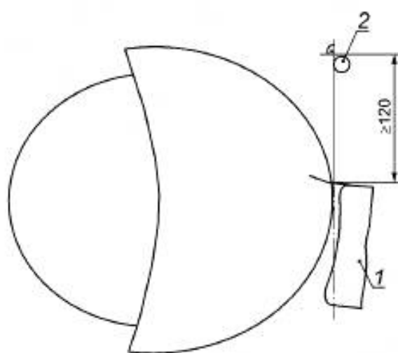
1 — глушитель; 2 — передняя рукоятка
