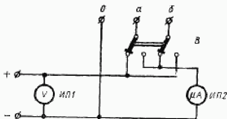
ИП1 — вольтметр постоянного тока; B — переключатель полярности напряжения; а и б — контакты, предназначенные для присоединения электродов, металлического баллона или подогревателя, между которыми измеряют сопротивление изоляции; в — контакт, являющийся общей точкой схемы; ИП2 — электронный или магнитоэлектрический микроамперметр постоянного тока.
