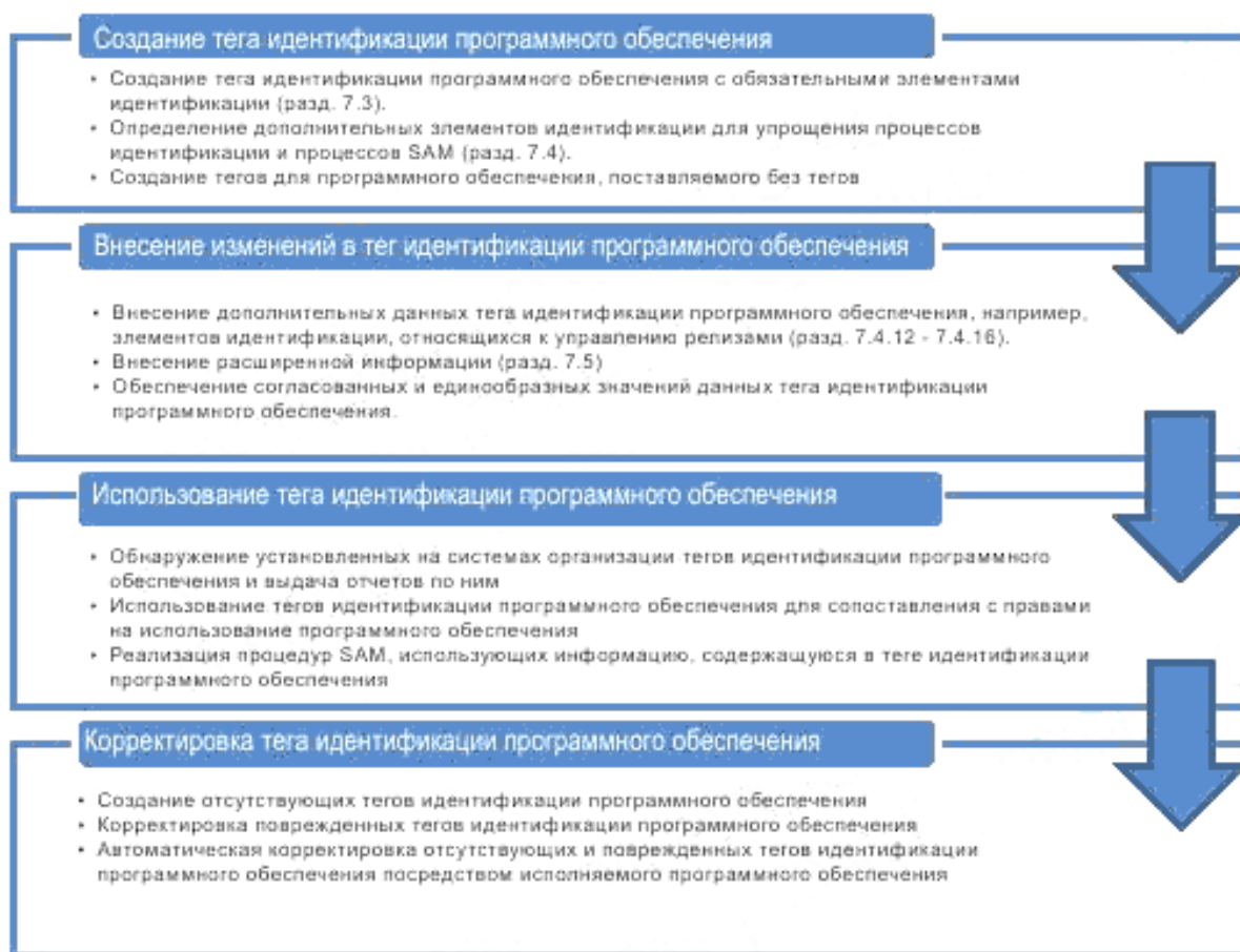
Рисунок 1 – Жизненный цикл работы с тегами идентификации программного обеспечения
